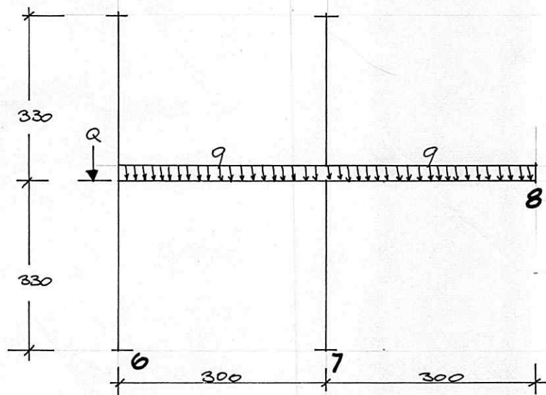
Schema di calcolo
