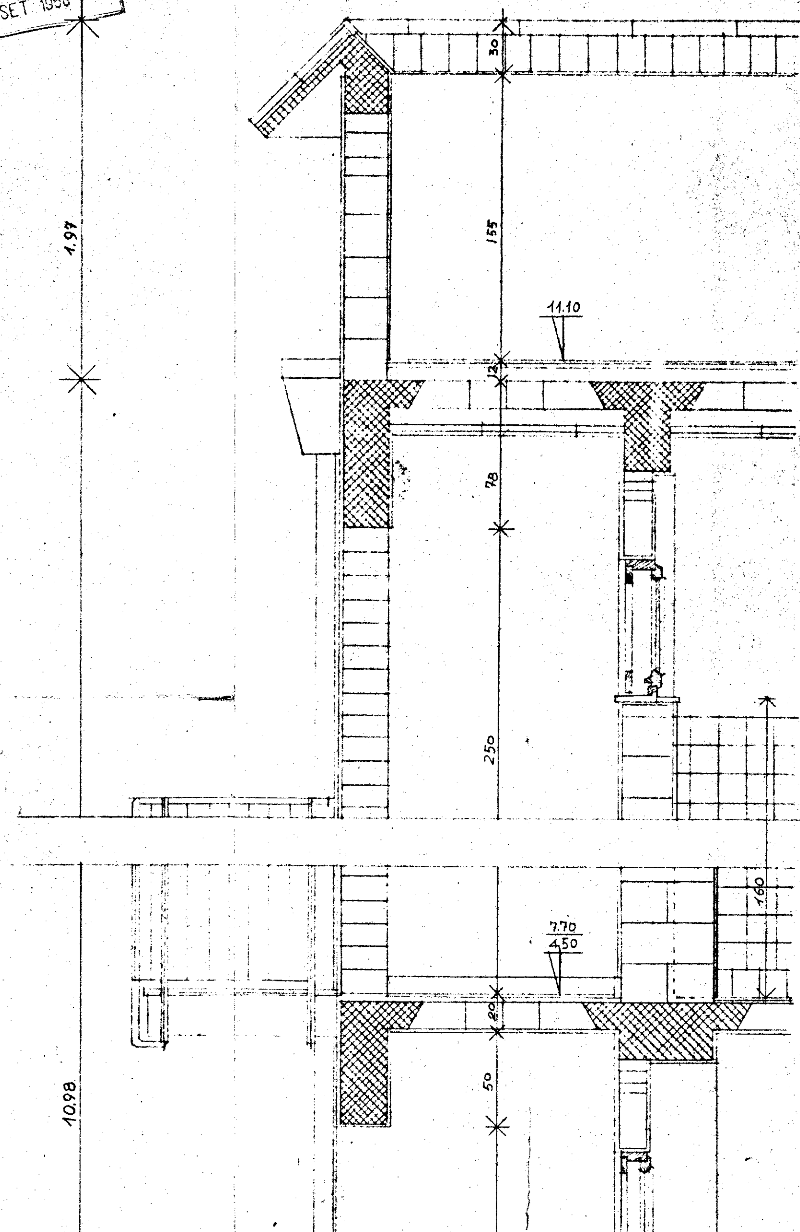
SEZ. D-D'
