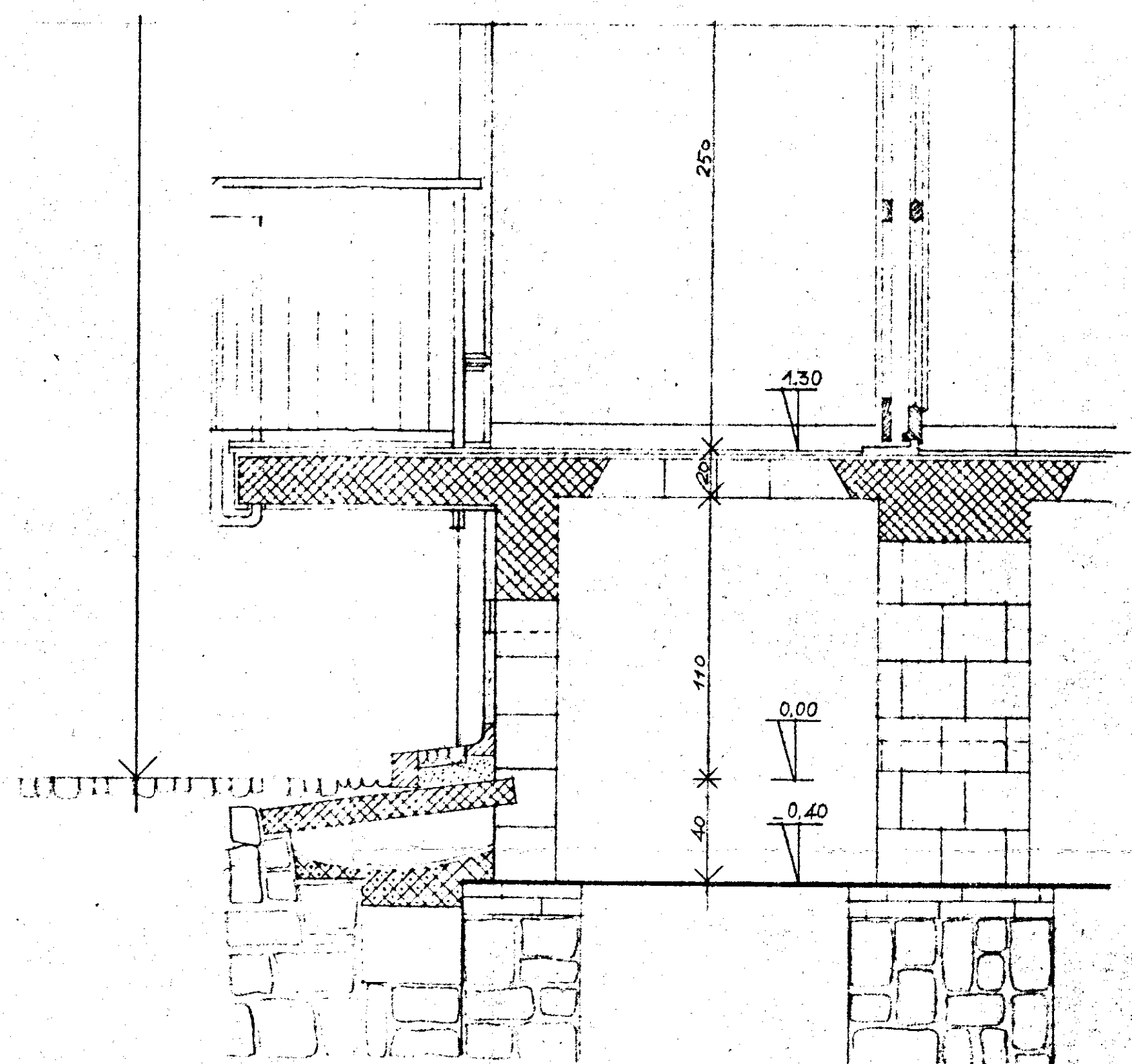
SEZ. C-C'
