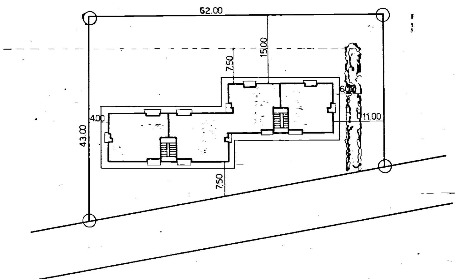
PLANIMETRIA GENERALE rapp. 1:500 AREA INTERVENTO GESCAL mq 2.400
