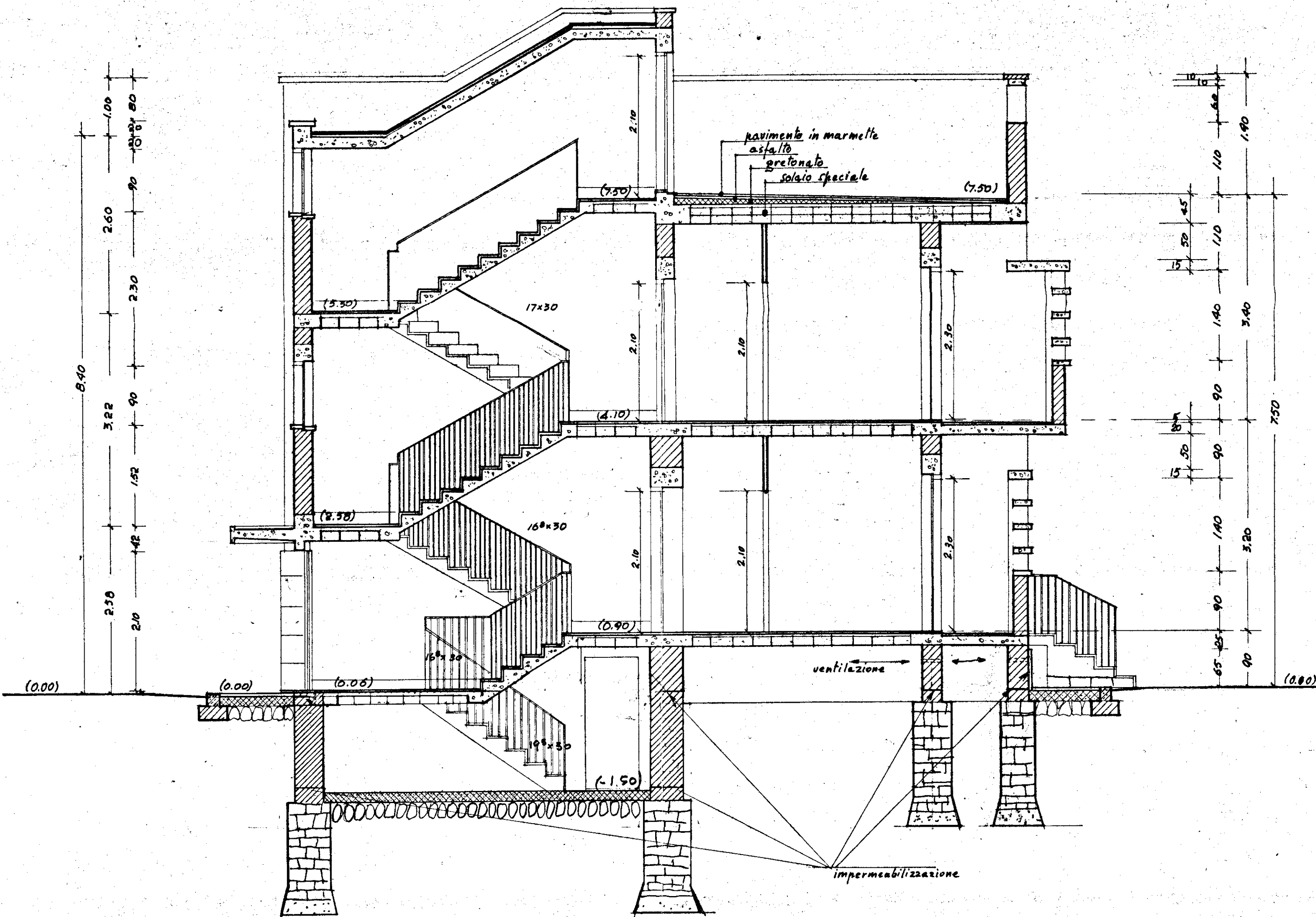
DIS. N° 197 SEZIONE A-B RAPP. 1:50
