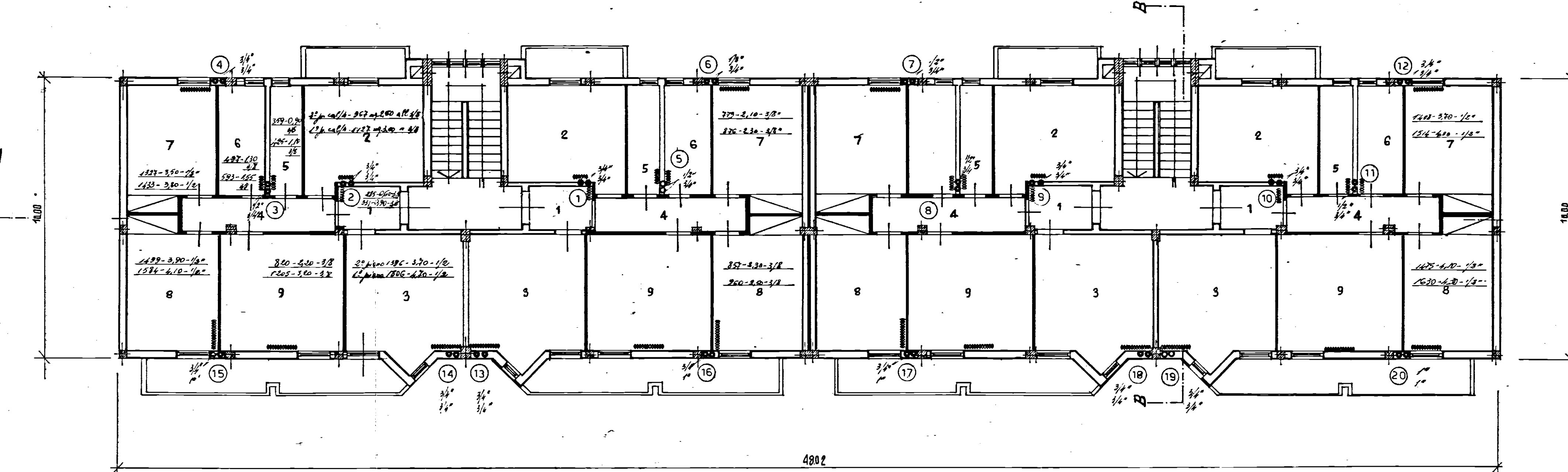
PIANTA 1° E 2° PIANO
