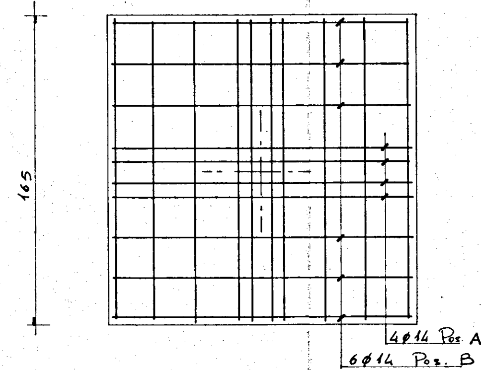
PLINTO C
