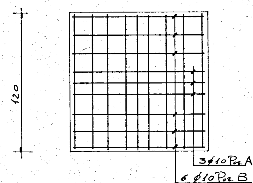
PLINTO A
