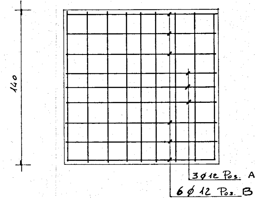
PLINTO B
