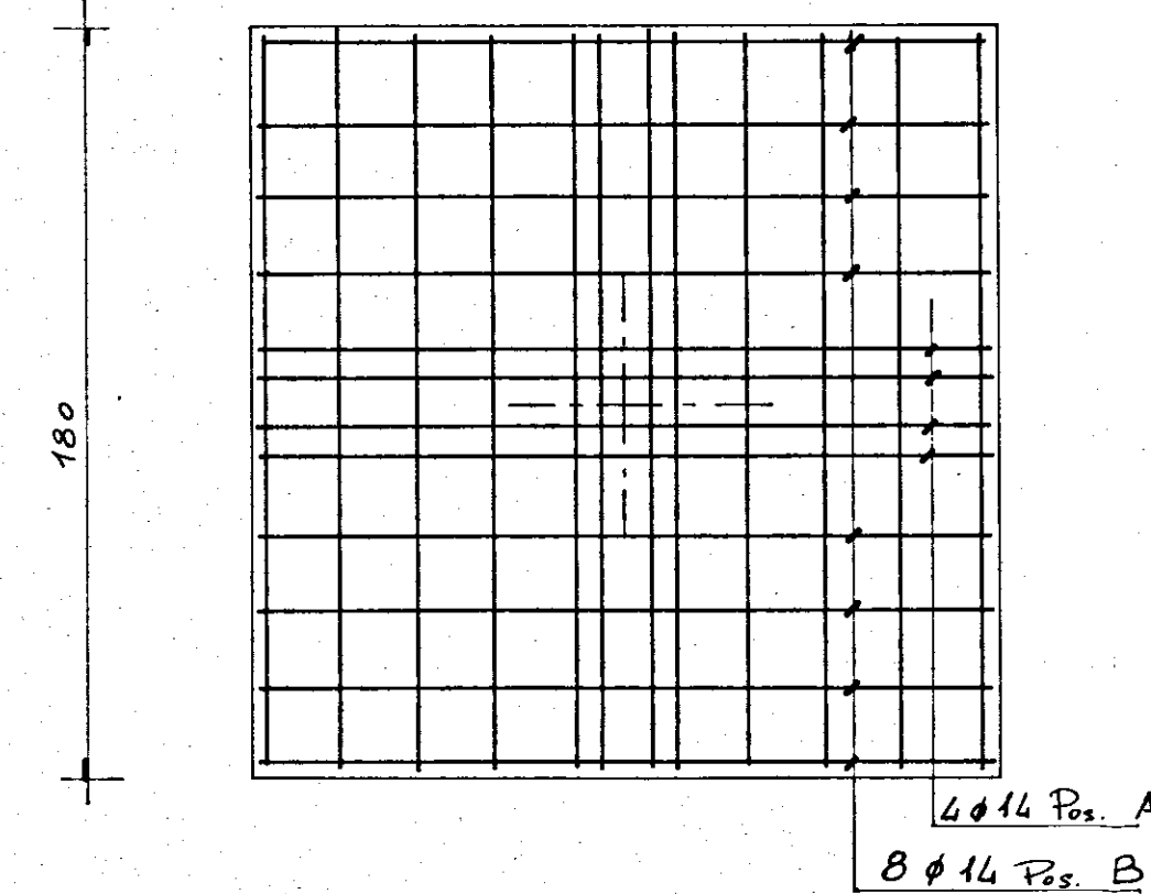
PLINTO D
