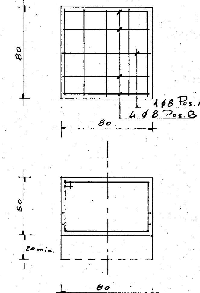
PLINTO F
