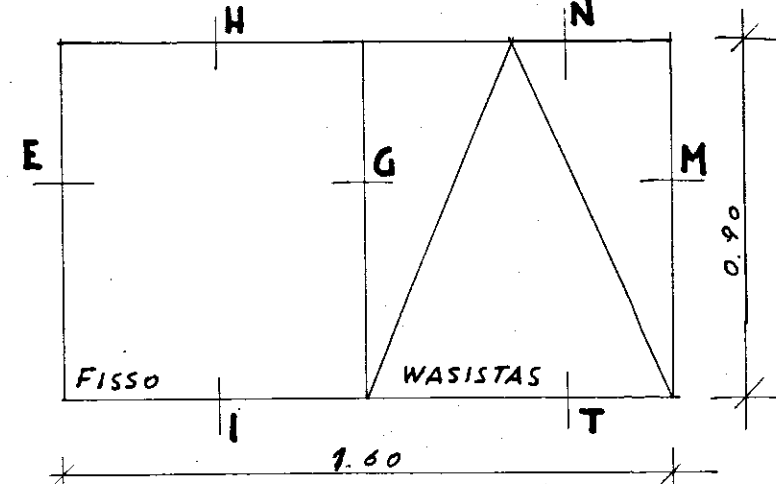
FINESTRA CON FISSO+WASISTAS, TIPO F7 PER SCALE
