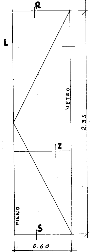
FINESTRA-PORTE TIPO F6 CON AVVOLGIBILE
