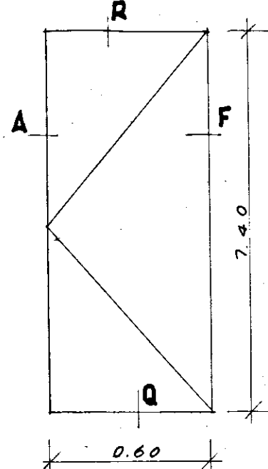
FINESTRA TIPO F5 CON AVVOLGIBILE
