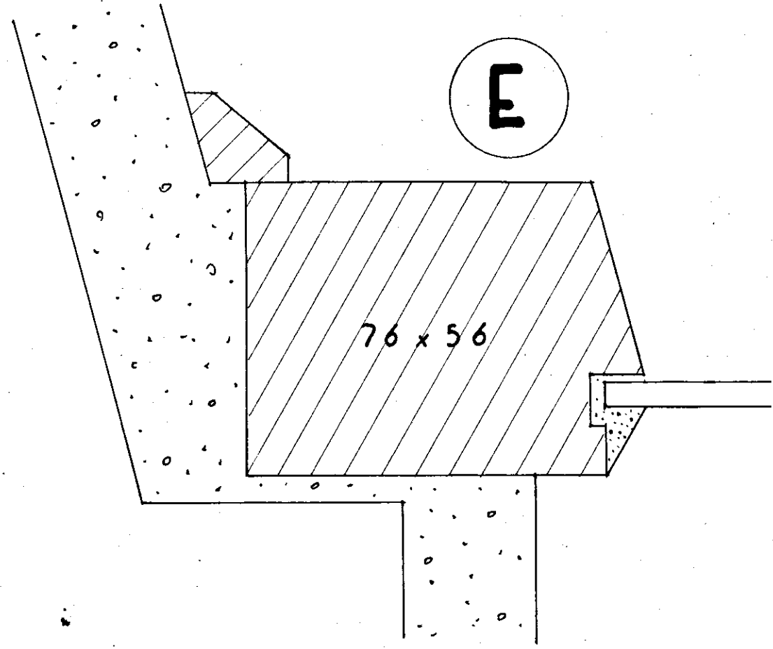
FINESTRA CON FISSO+WASISTAS, TIPO F7 PER SCALE
