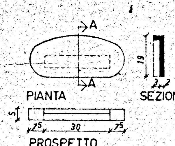
PIANTA
