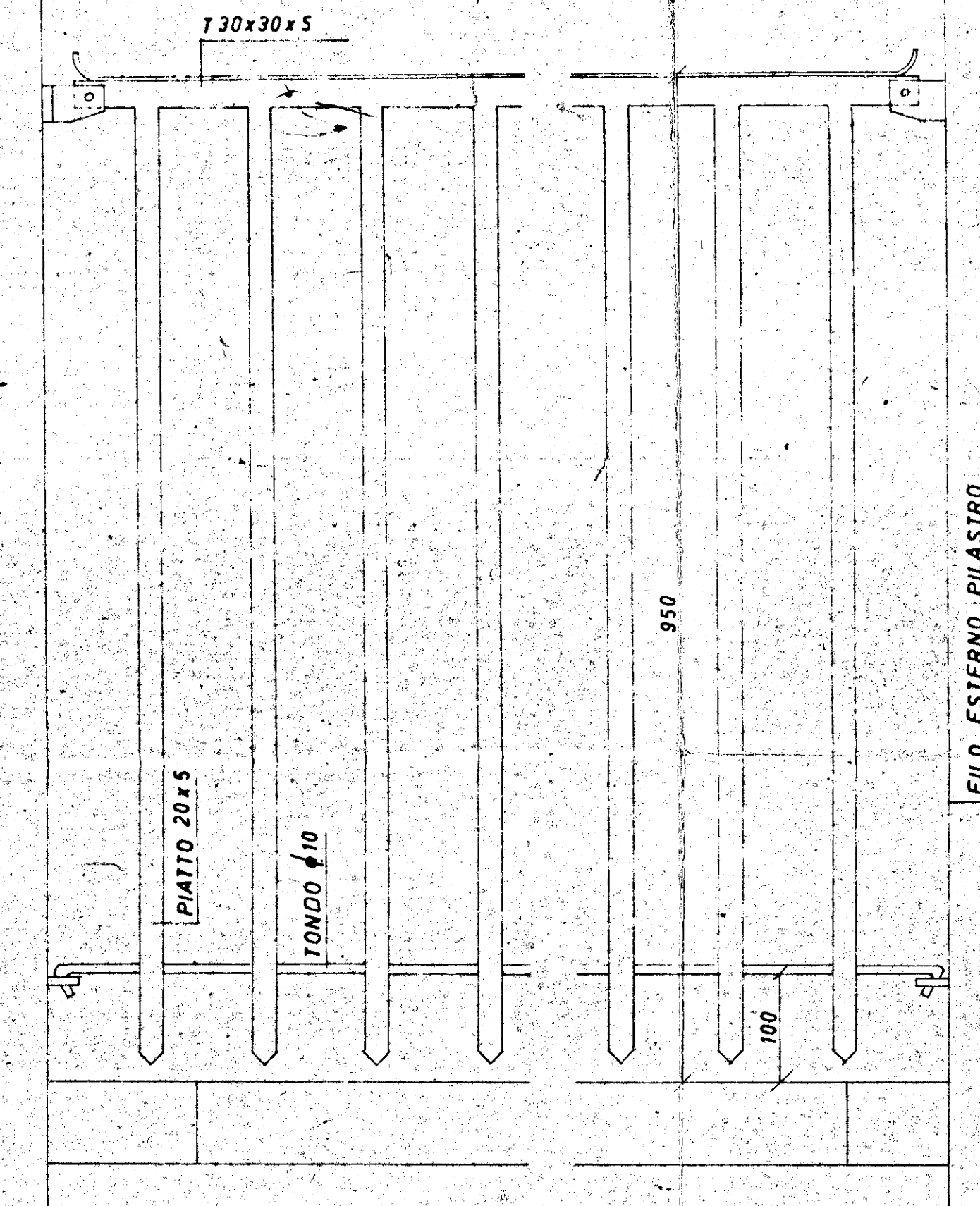
PROSPETTO
