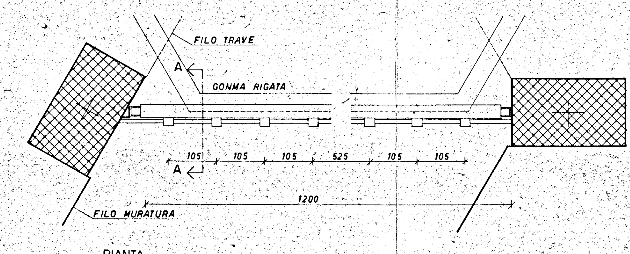
PIANTA
