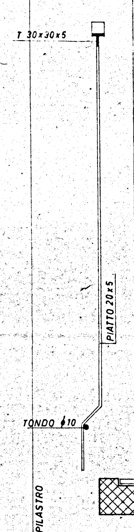
SEZIONE A-A
