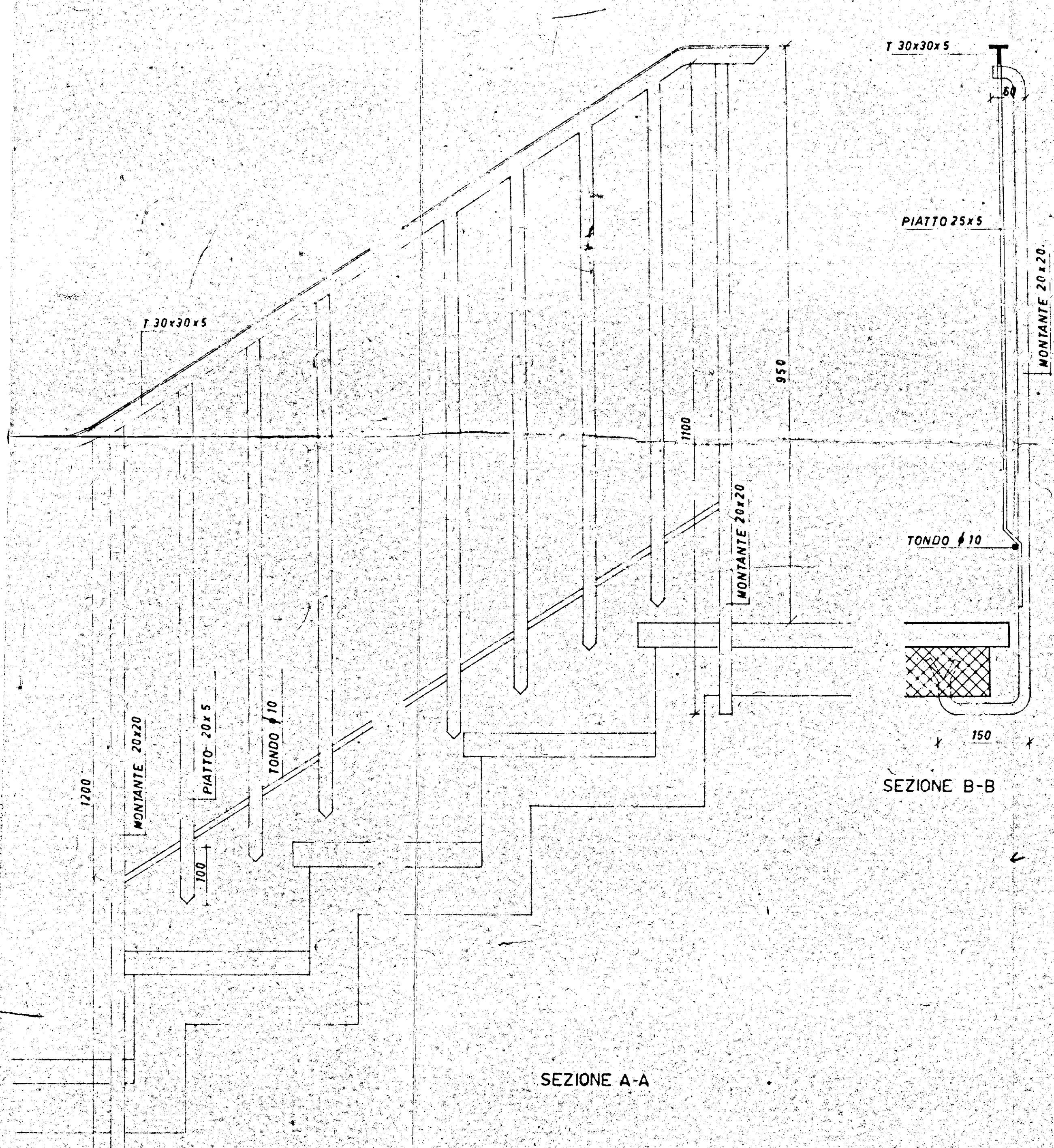
RINGHIERA SCALA RAPP.1:5
