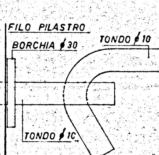
SEZIONE A-A
