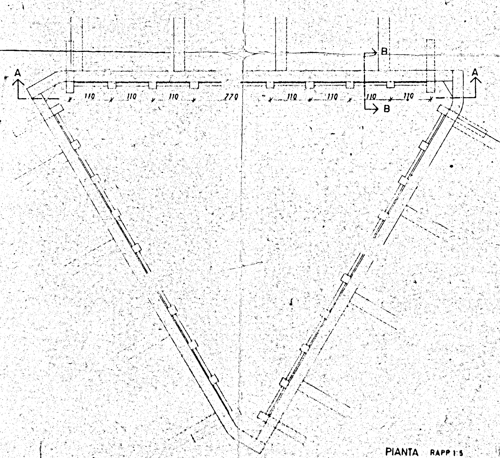
PIANTA RAPP.1:5
