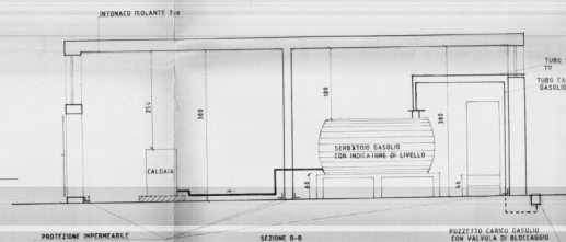
SEZIONE B-B
