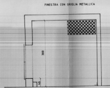
SEZIONE C-C
