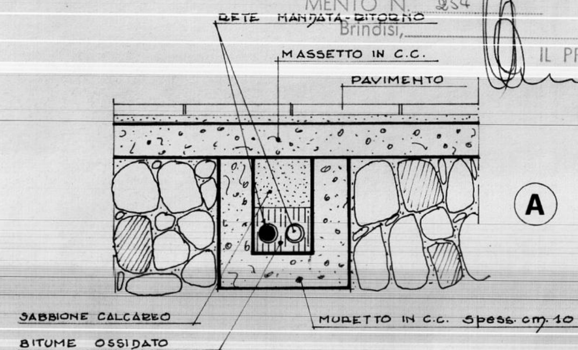
PARTICOLARE RETE INTERRATA IN CUNICOLO - Rapp. 1/10
