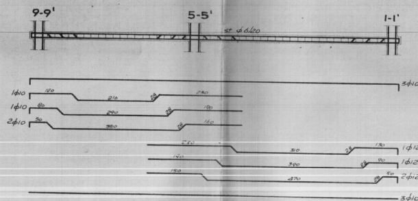
SEZIONE GENERICA TRAVE
