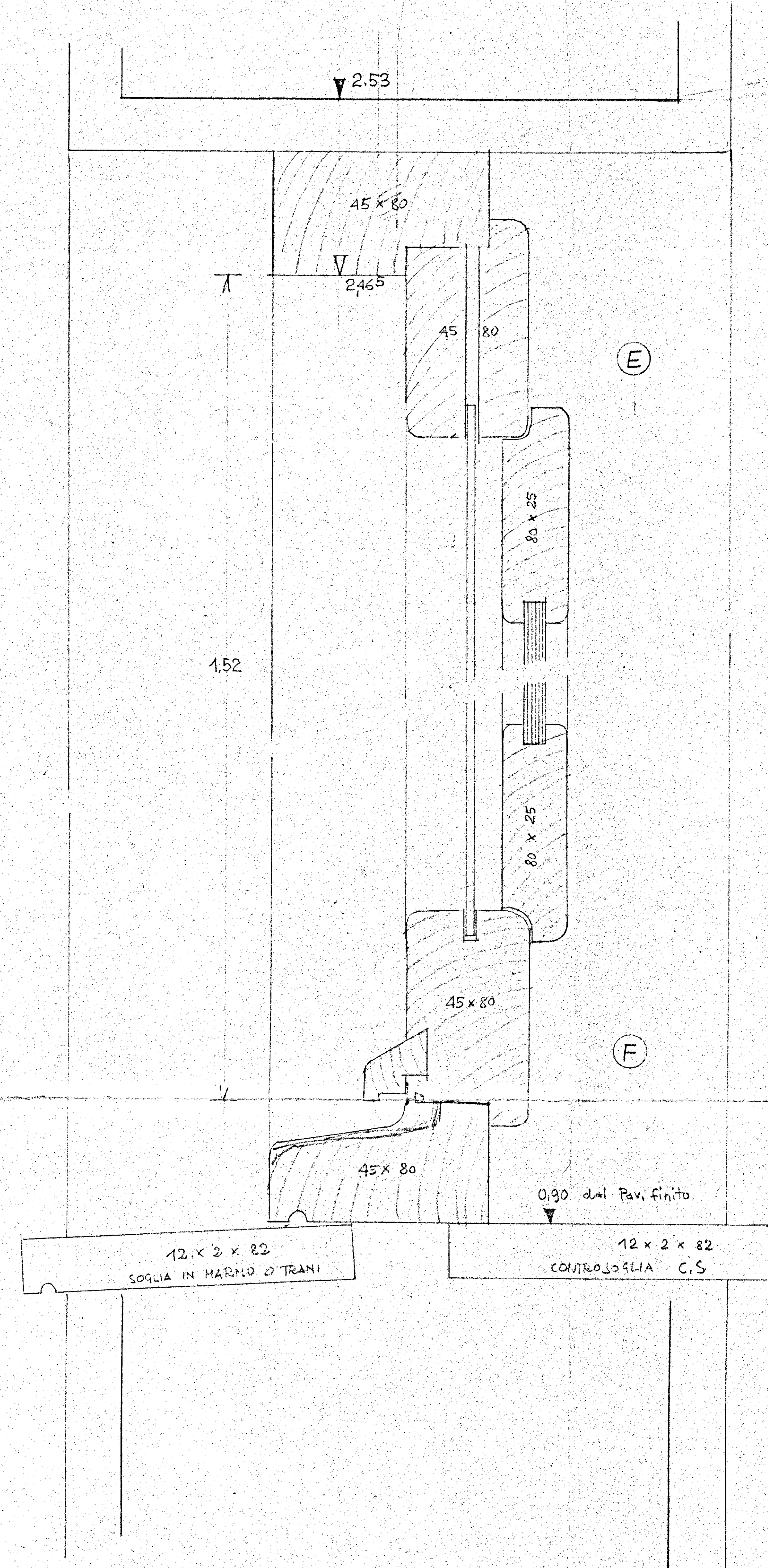
F FINESTRE DEI BAGNI N° 32 CON SCURETTI PILATO STAMPATO 63 x 141
