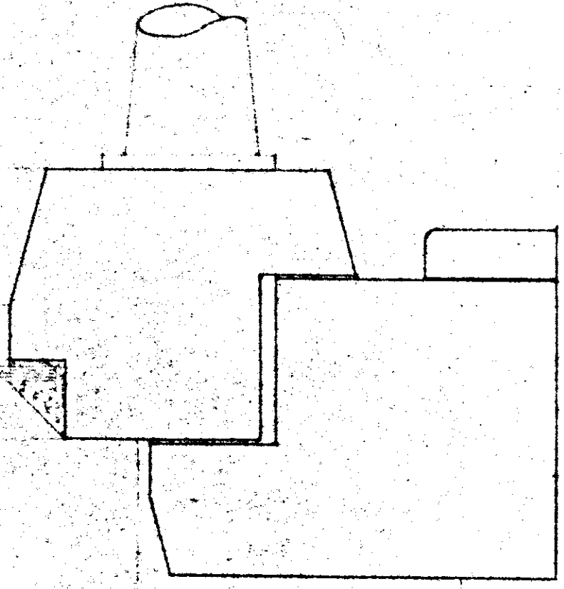
SEZIONE 4 TAV. 8
