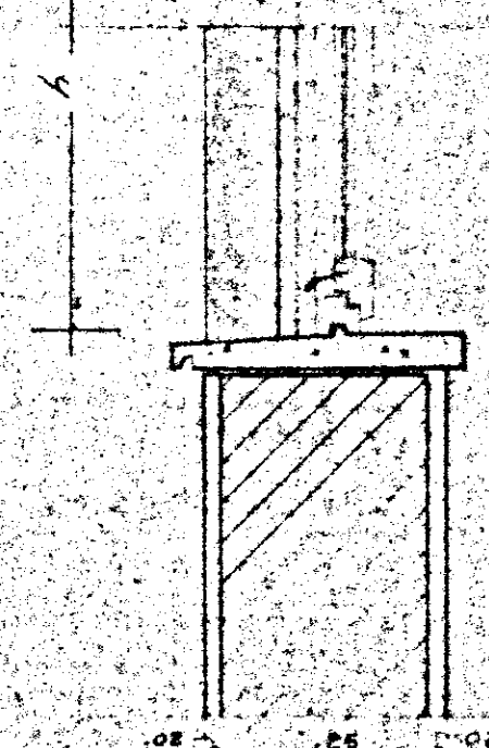
SEZIONE TIPO
