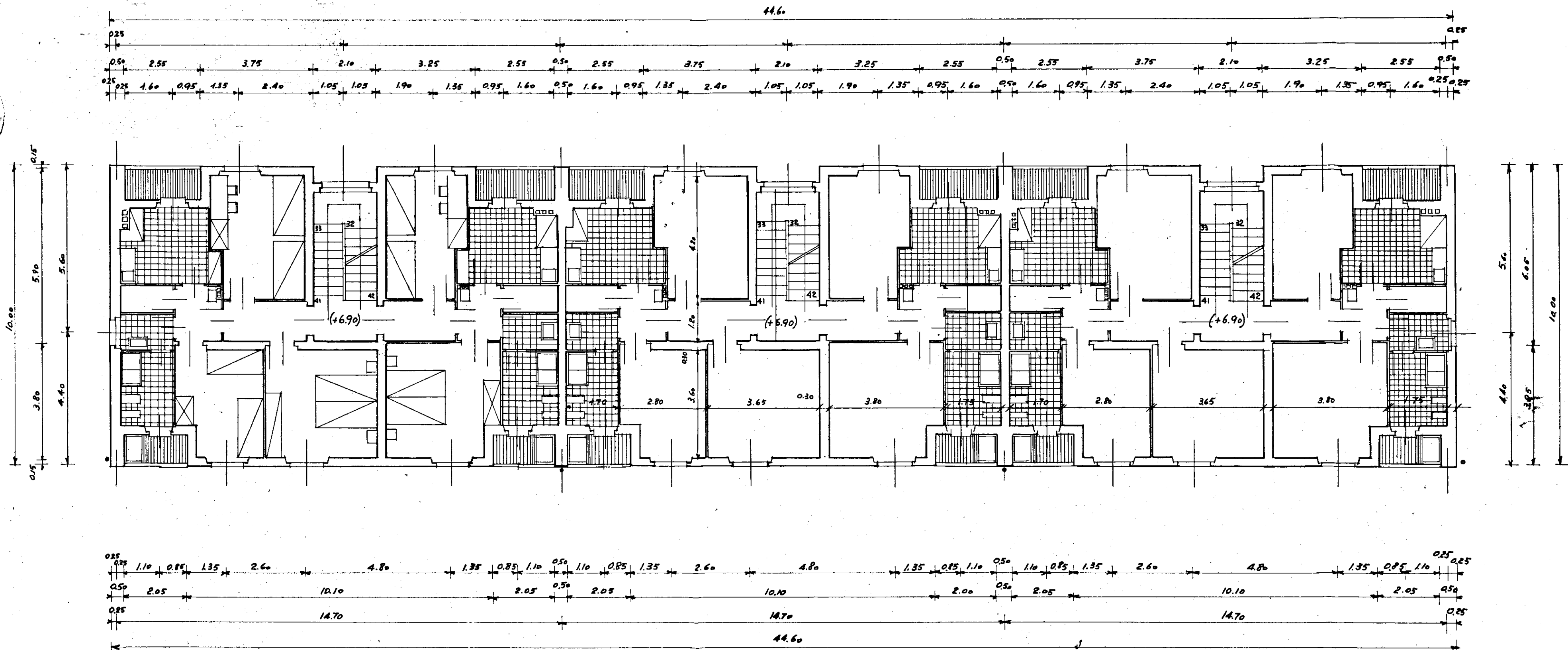
DIS. N° 95 PIANA 2° PIANO (TIPO - 1° e 2°)
