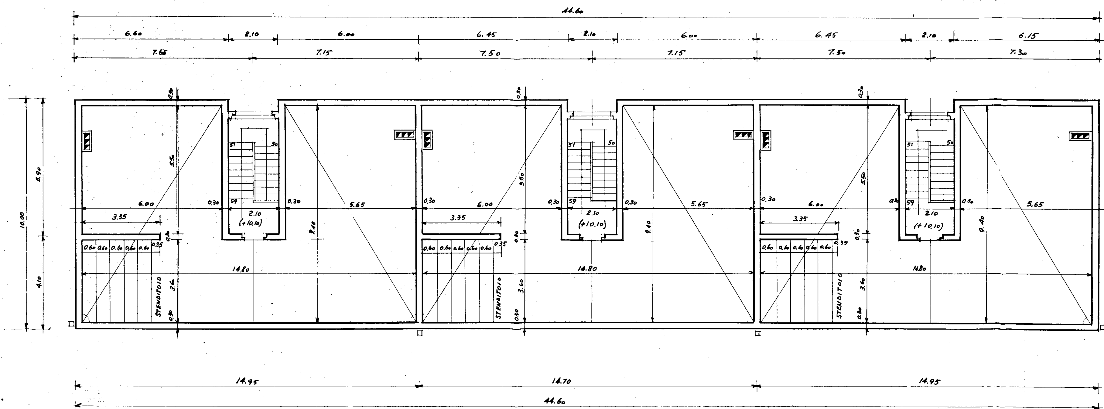
DIS. N° 96 PIANA COPERTURA
