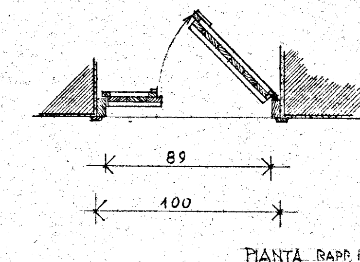
PIANTA RAPP. 1:20
