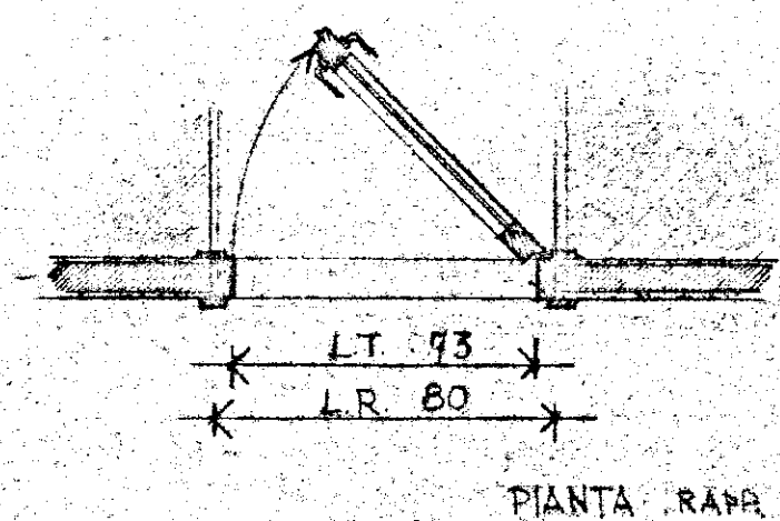
PIANTA RAPP. 1:20
