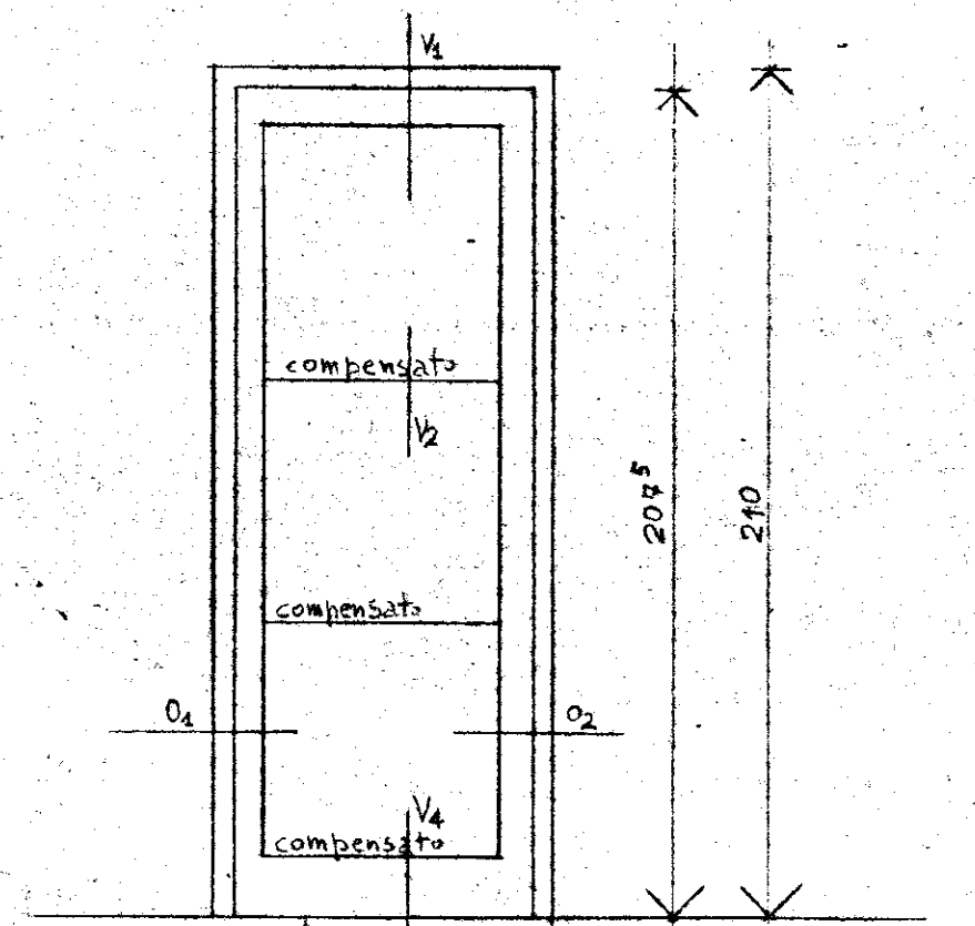
TIPO B BUSSOLA AD UNA PARTITA RAPP. 1:20
