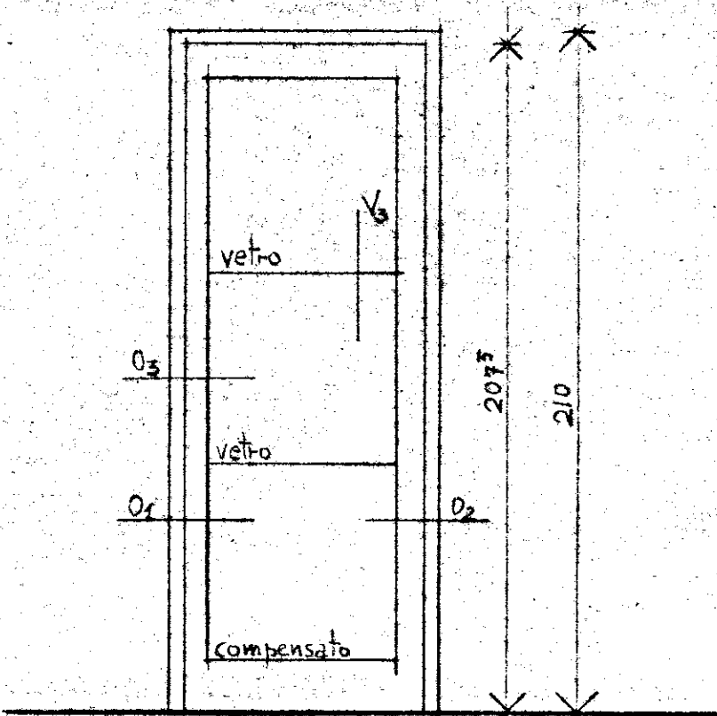
TIPO A BUSSOLA AD UNA PARTITA CON SPECCHIO A VETRI RAPP. 1:20
