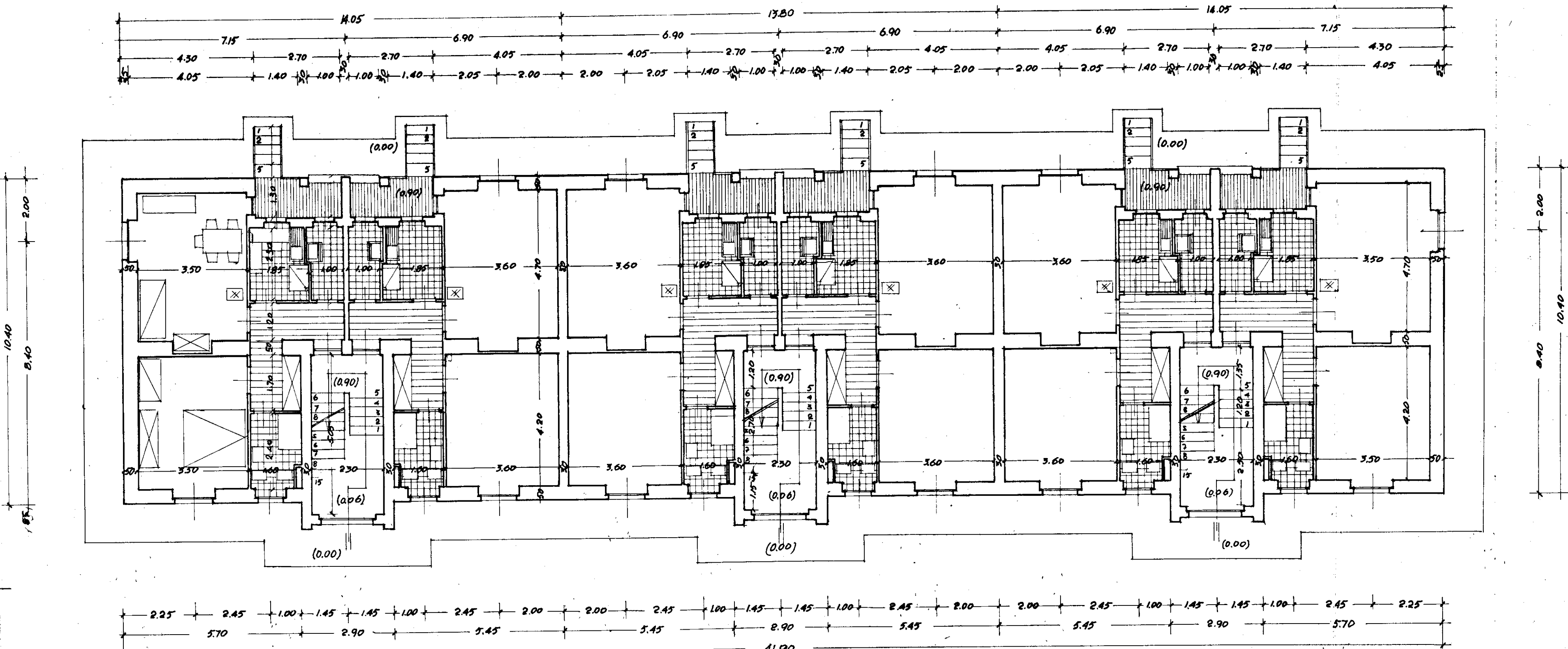
DIS. N° 187 PIANO RIALZATO RAPP. 1:100
