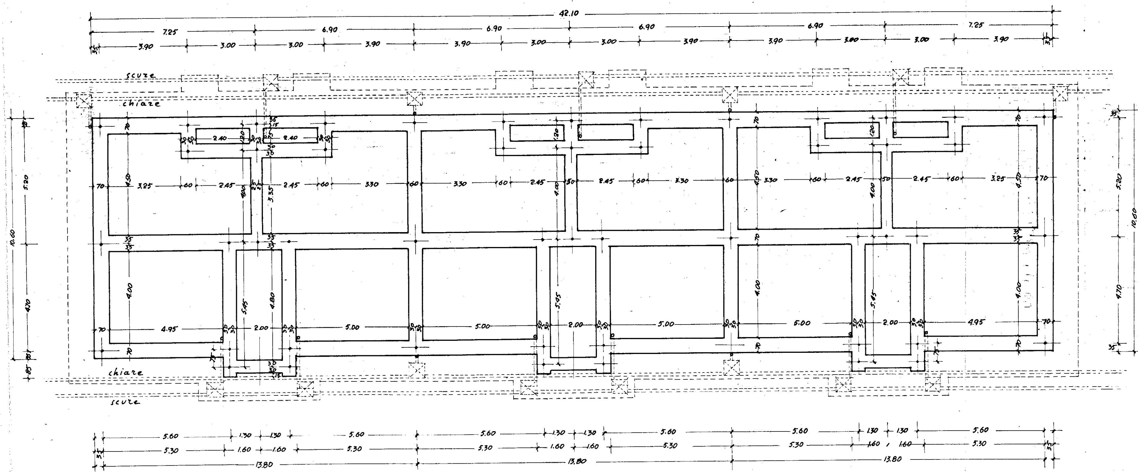
DIS. N° 186 FONDAZIONE E SCHEMA FOGNE RAPP. 1:100
