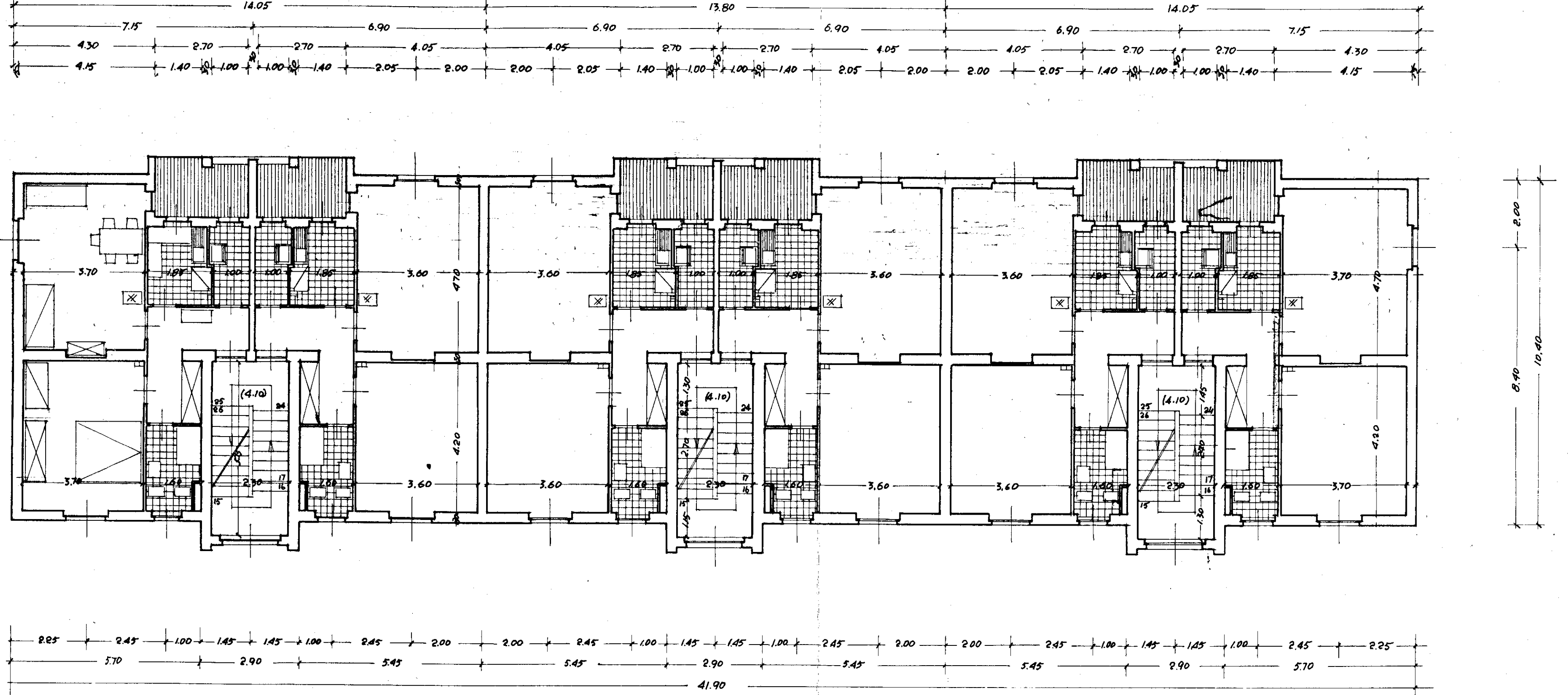
DIS. N° 188 PRIMO PIANO RAPP. 1:100
