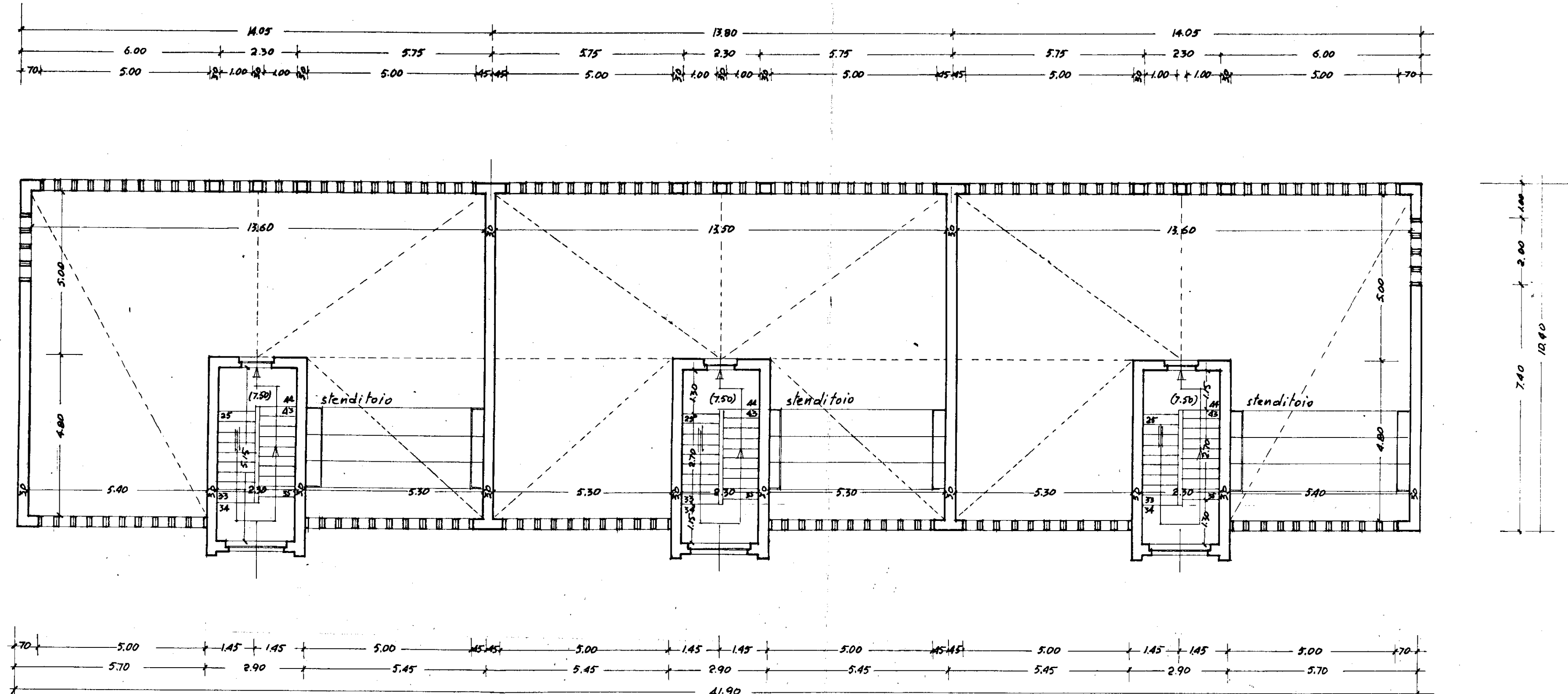
DIS. N° 189 TERRAZZA DI COPERTURA RAPP. 1:100
