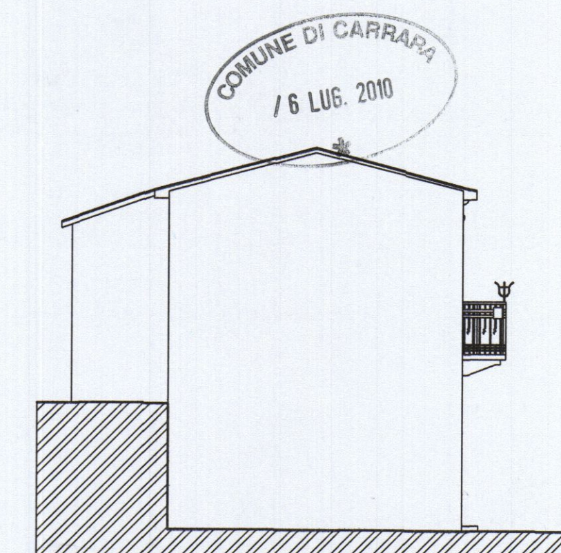
PROSPETTO OVEST
