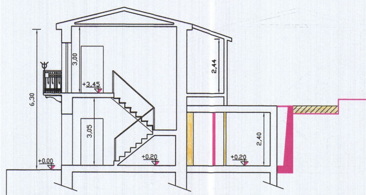
SEZIONE A-A'
