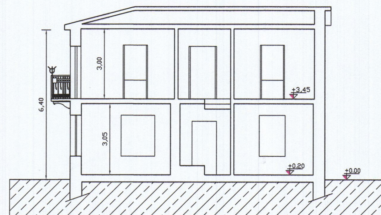
SEZIONE B-B'
