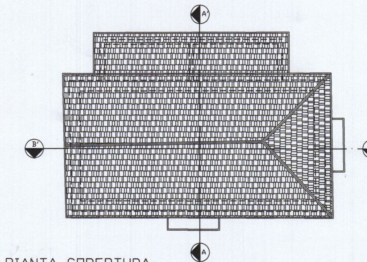
PIANTA COPERTURA
