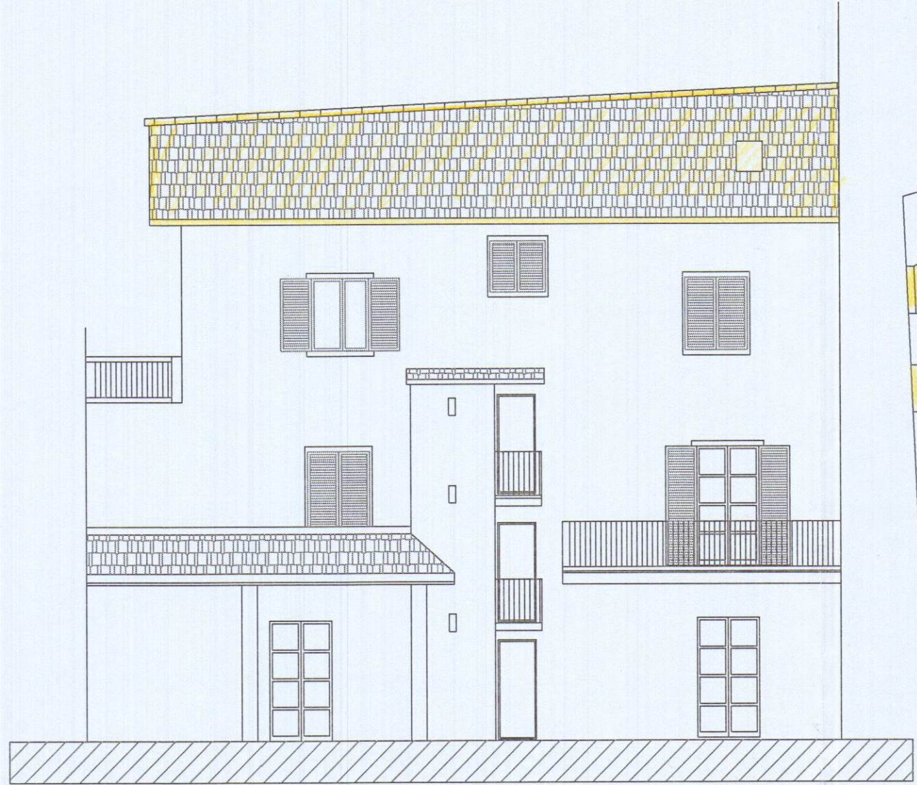
PROSPETTO SUD
