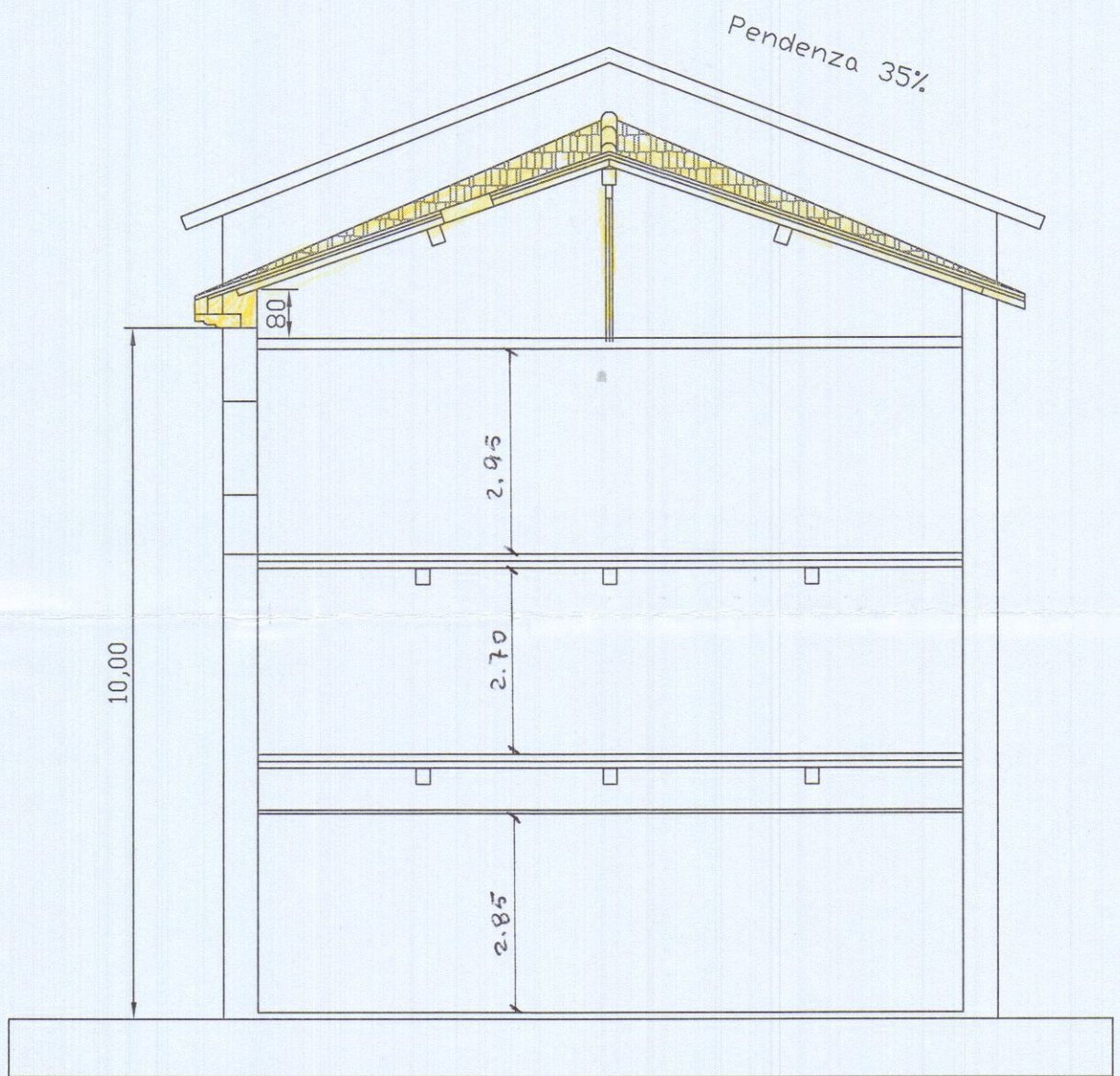
SEZ. A-A
