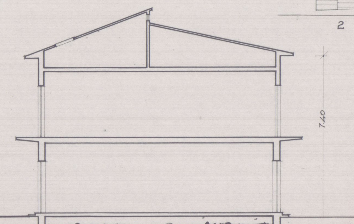
SEZIONE A-A.
