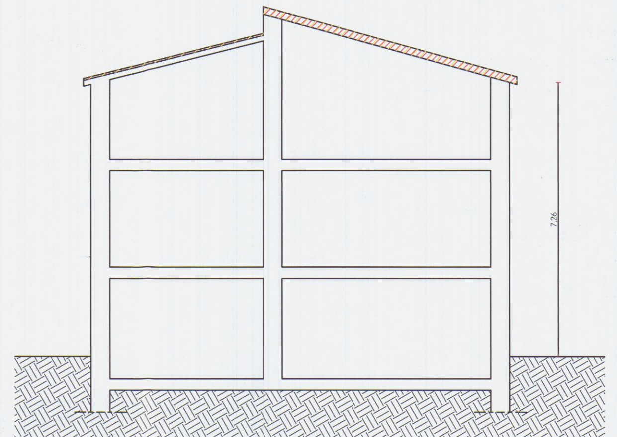
SEZIONE A-A
