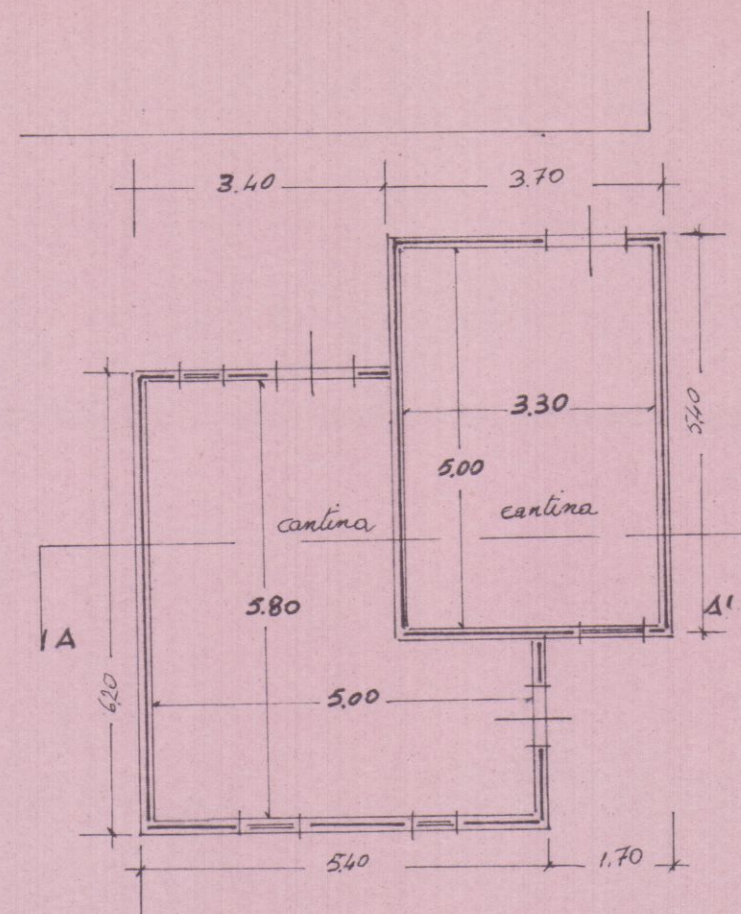
PIANTA
