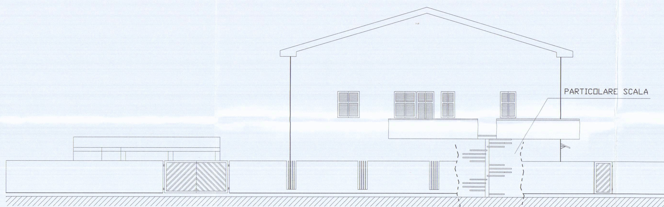
PROSPETTO NORD-OVEST
