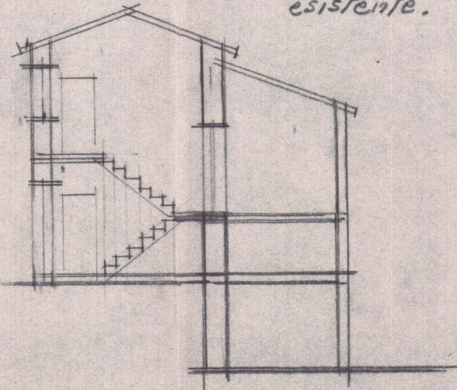
Sezione B-B' esistente.
