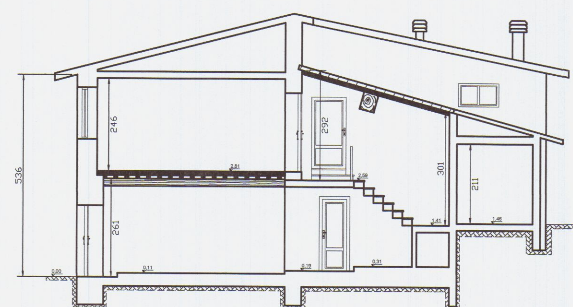
SEZIONE A-A
