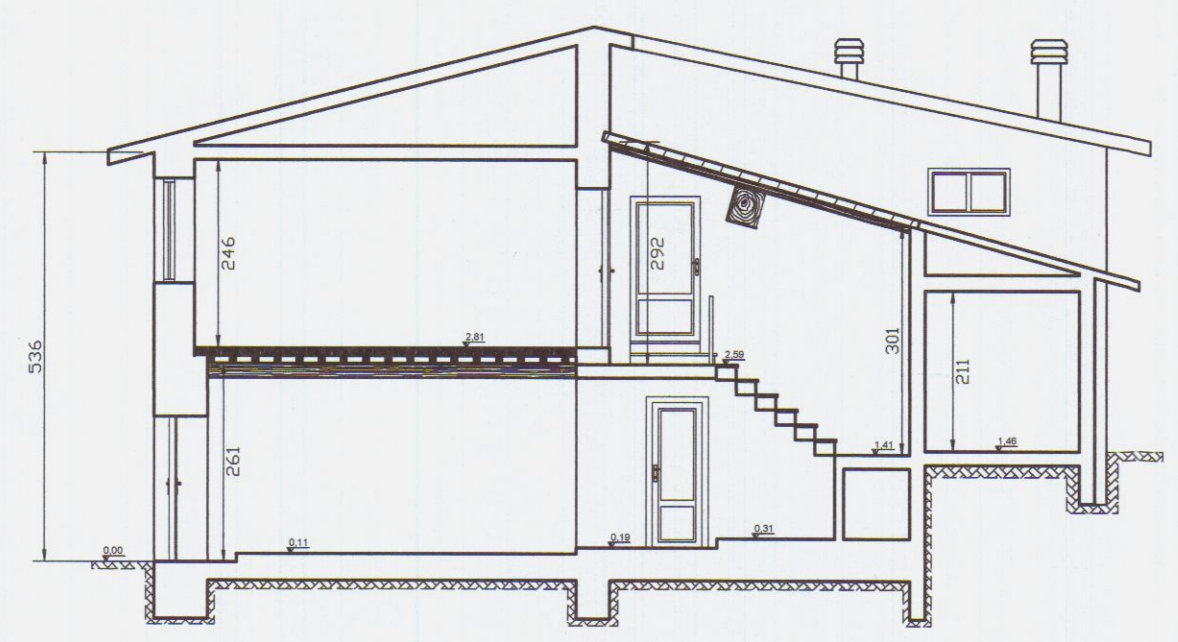
SEZIONE A-A
