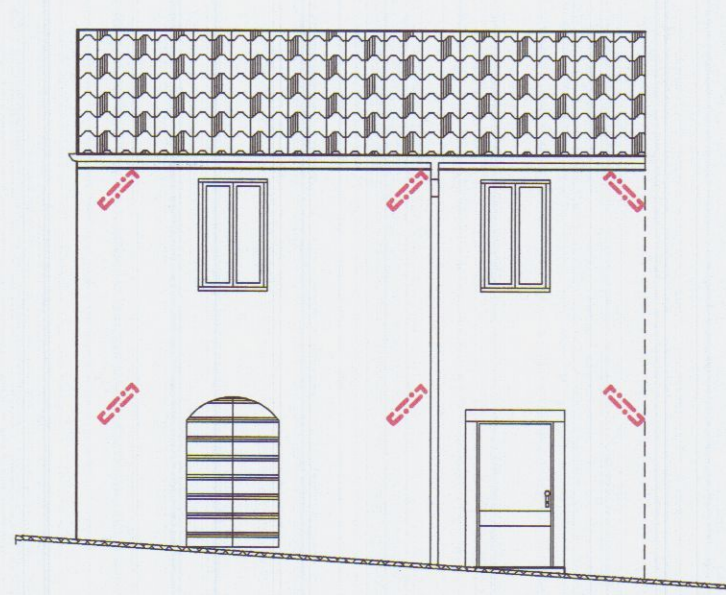
PROSPETTO LATO MARE
