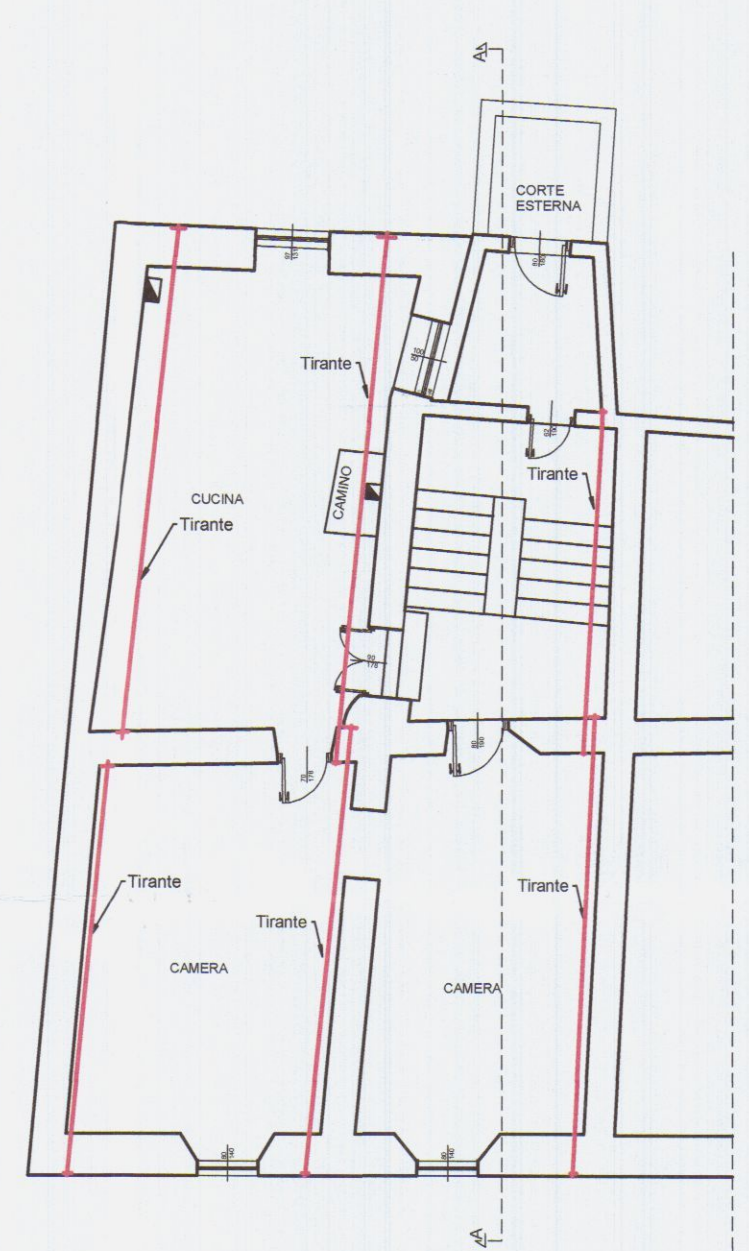
PIANO PRIMO
