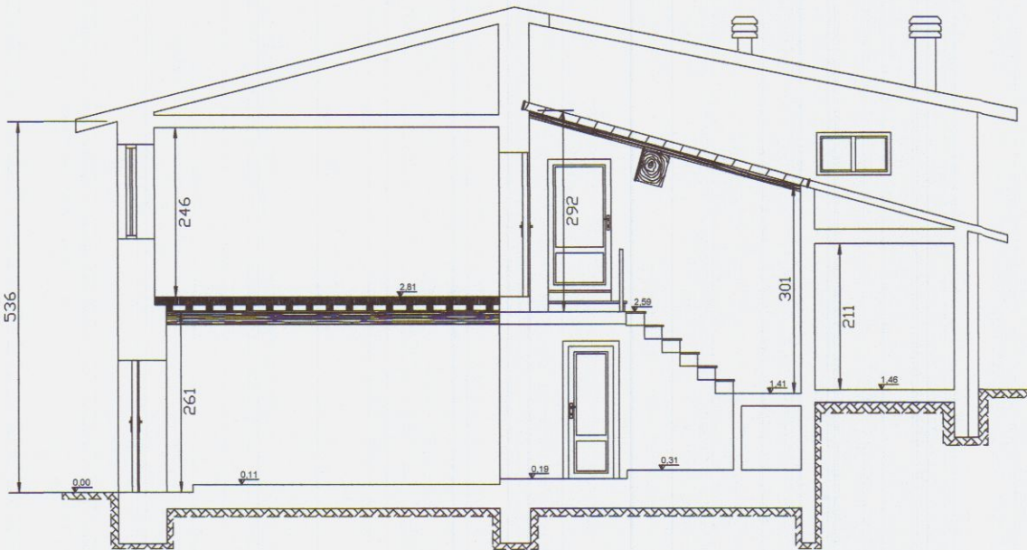
SEZIONE A-A
