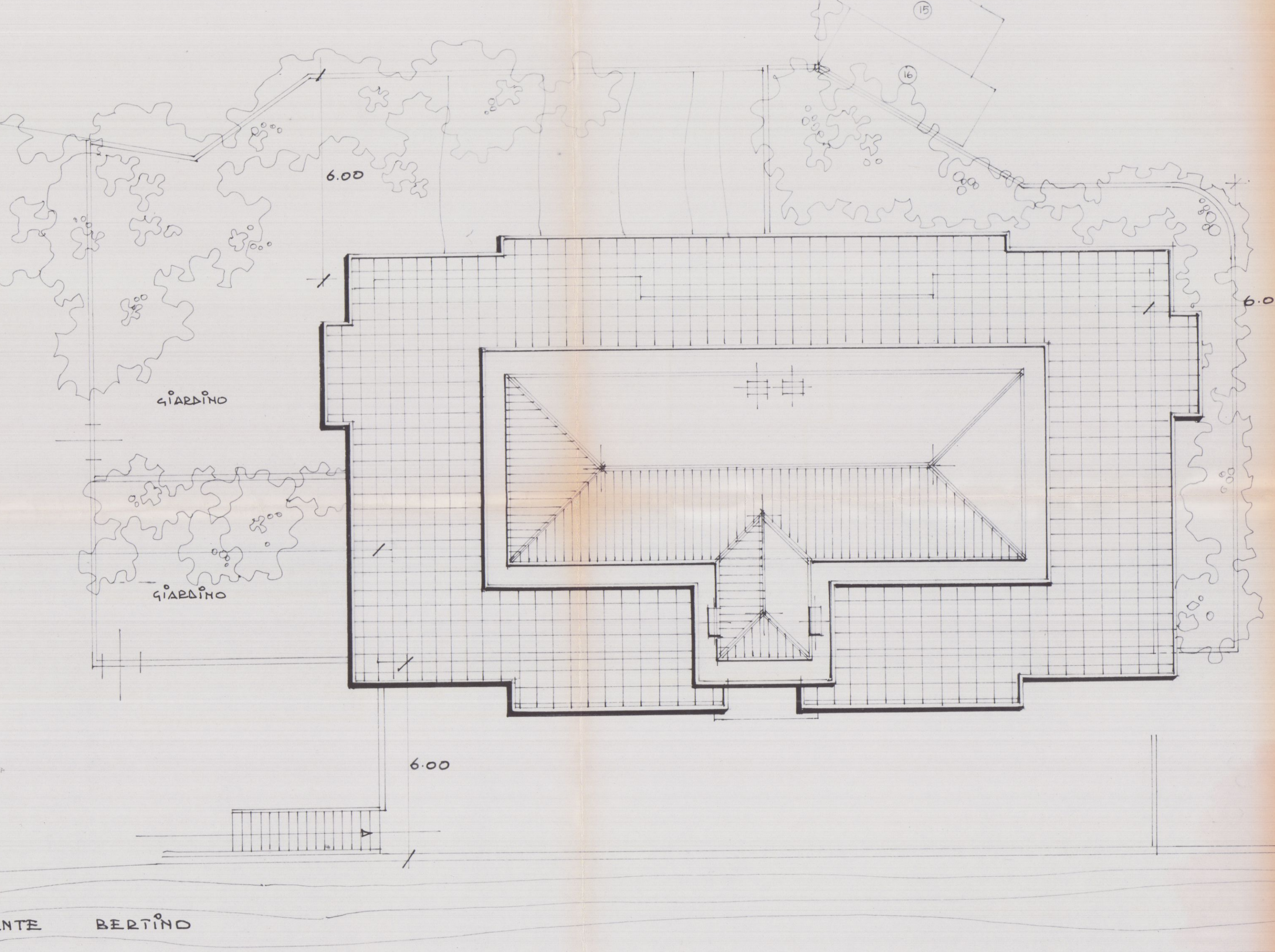
PIANTA COPERTURA E SISTEMAZIONE ESTERNA SCALA 1:100
