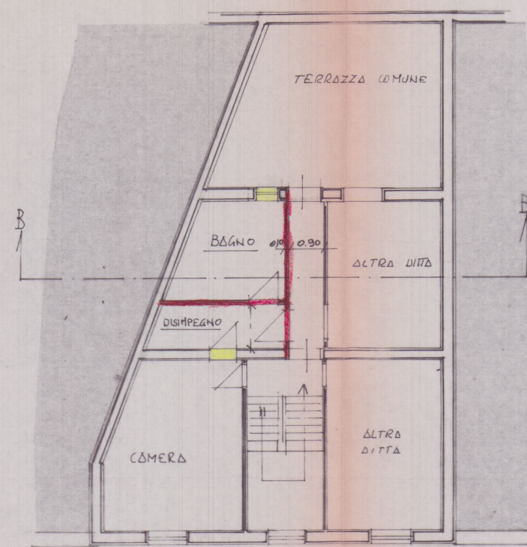
PIANO PRIMO
