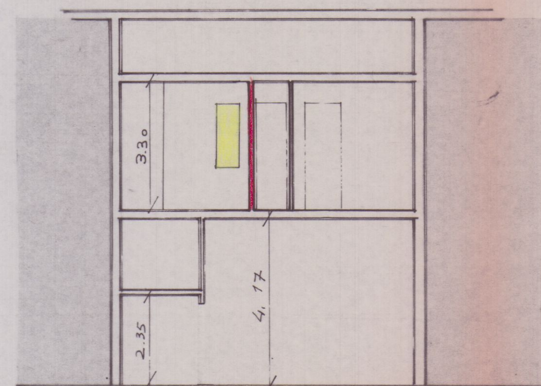
SEZIONE B-B
