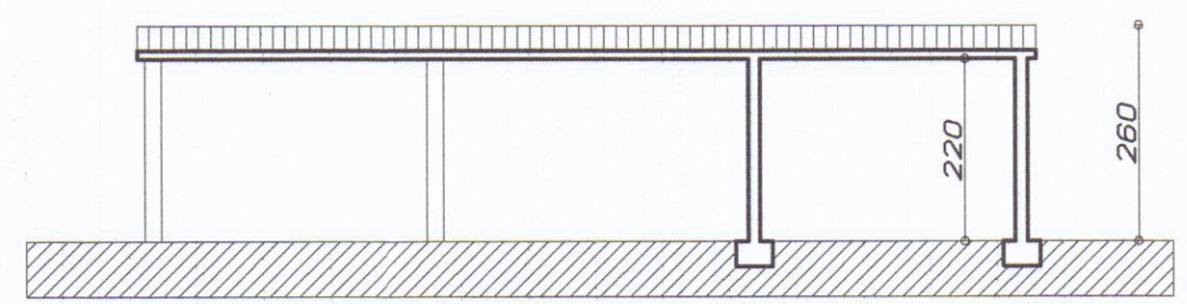
SEZIONE A.A.
