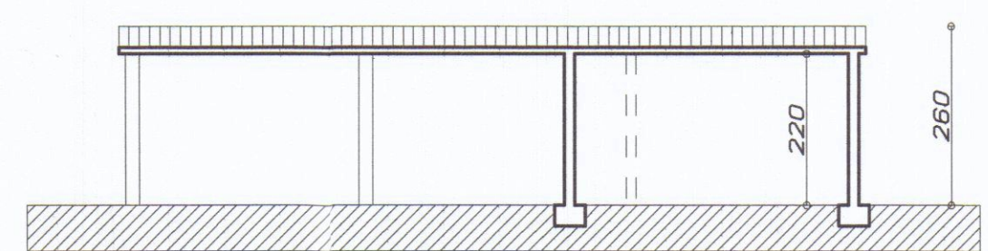
SEZIONE A.A.
