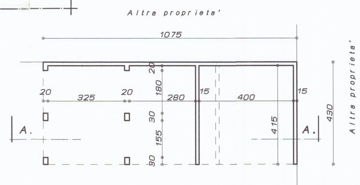
PIANTA
