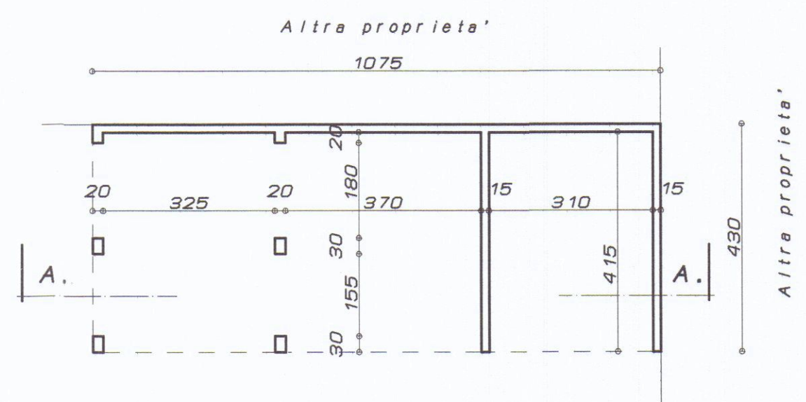
PIANTA
