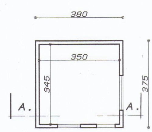
PIANTA
