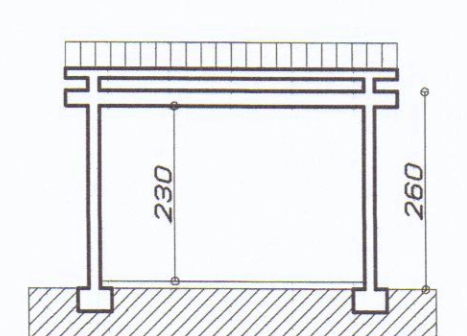
SEZIONE A.A.
