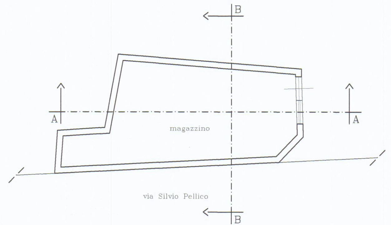
PIANTA INTERRATO
