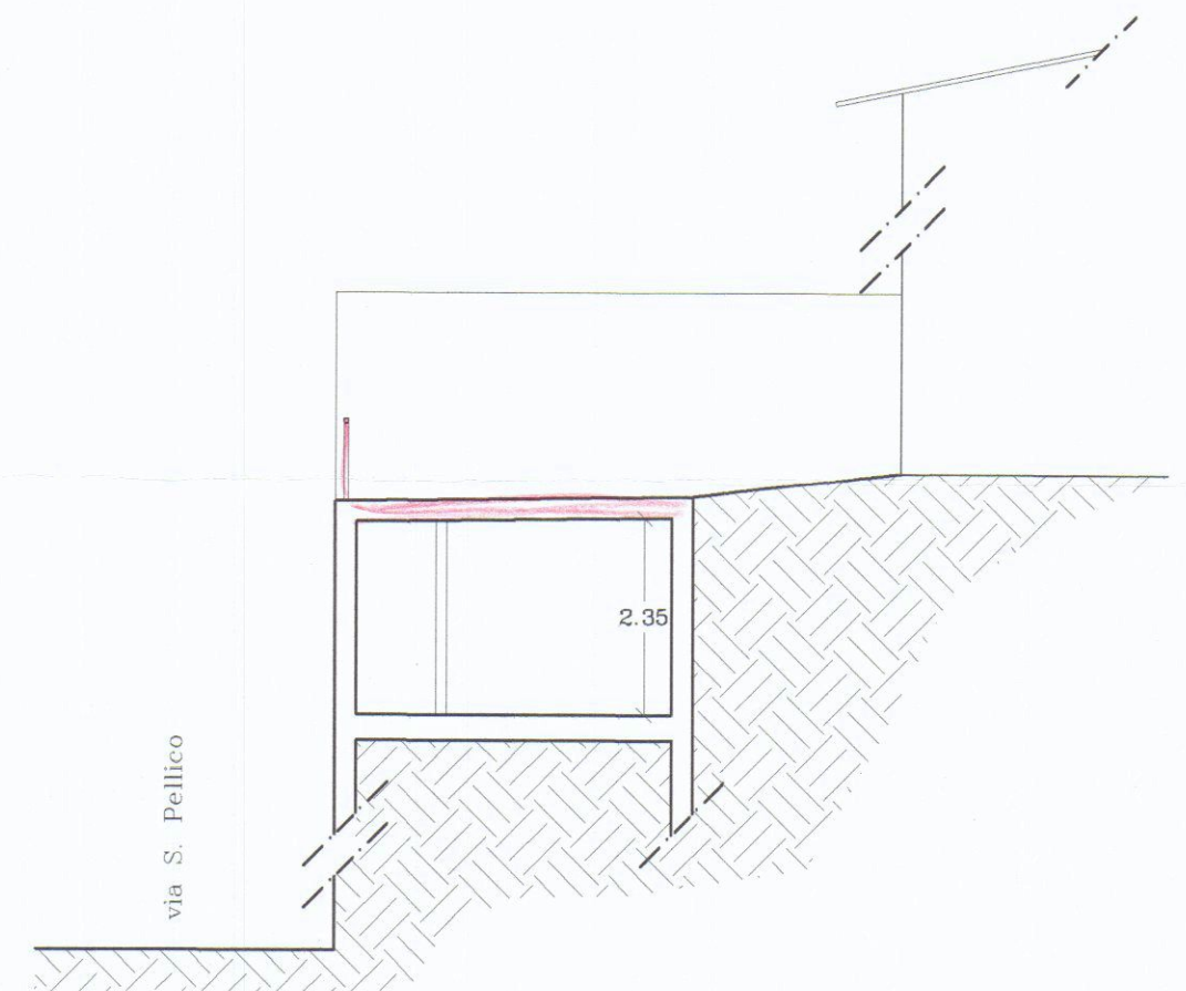
SEZIONE B - B
