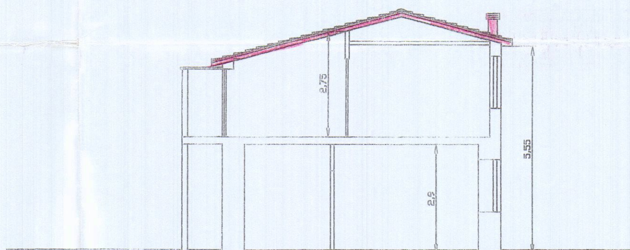
SEZIONE
