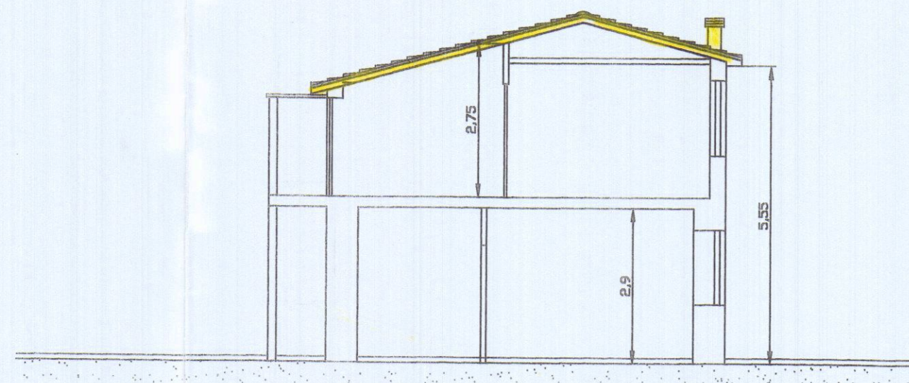
SEZIONE
