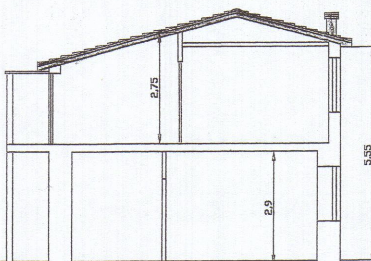
SEZIONE
