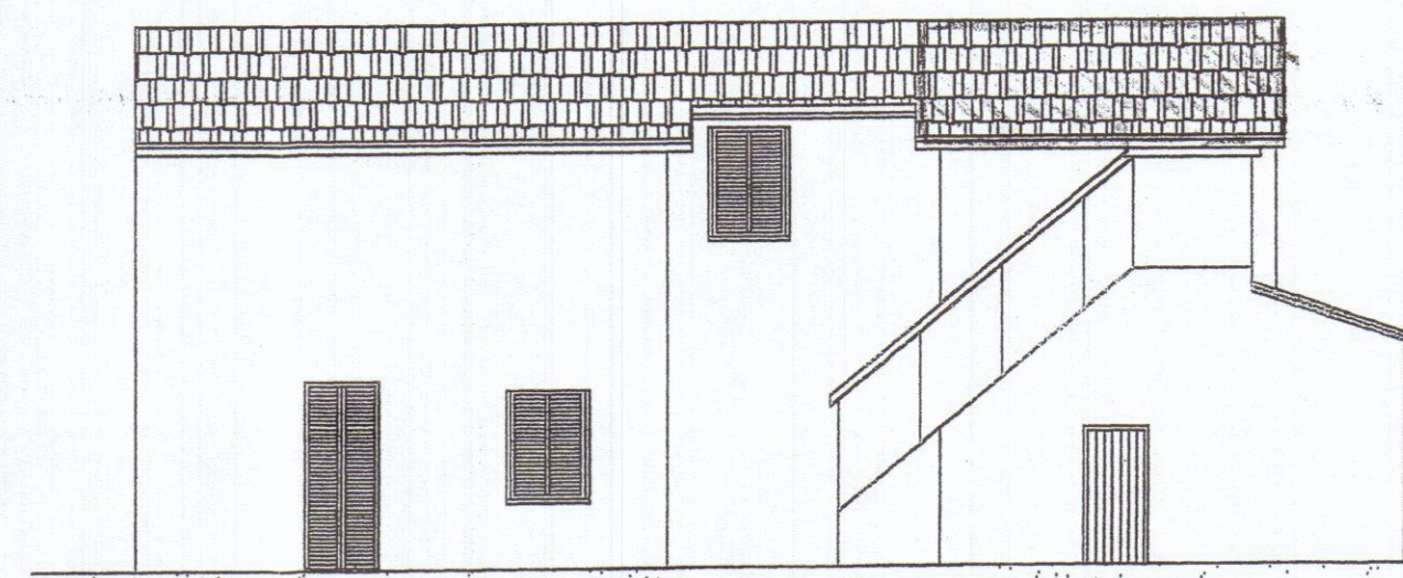
PROSPETTO SUD
