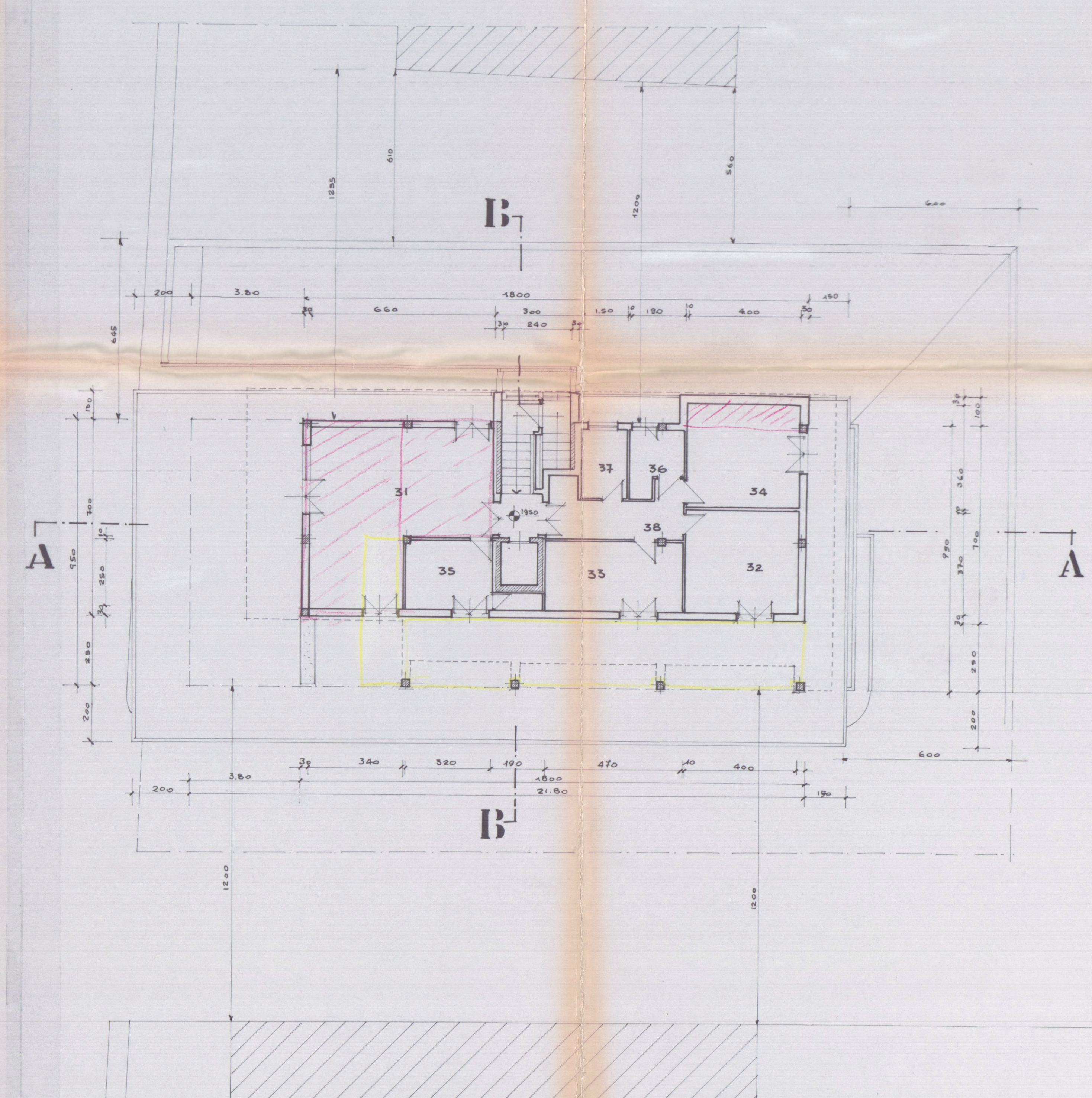
PIANTA PIANO ATTICO
