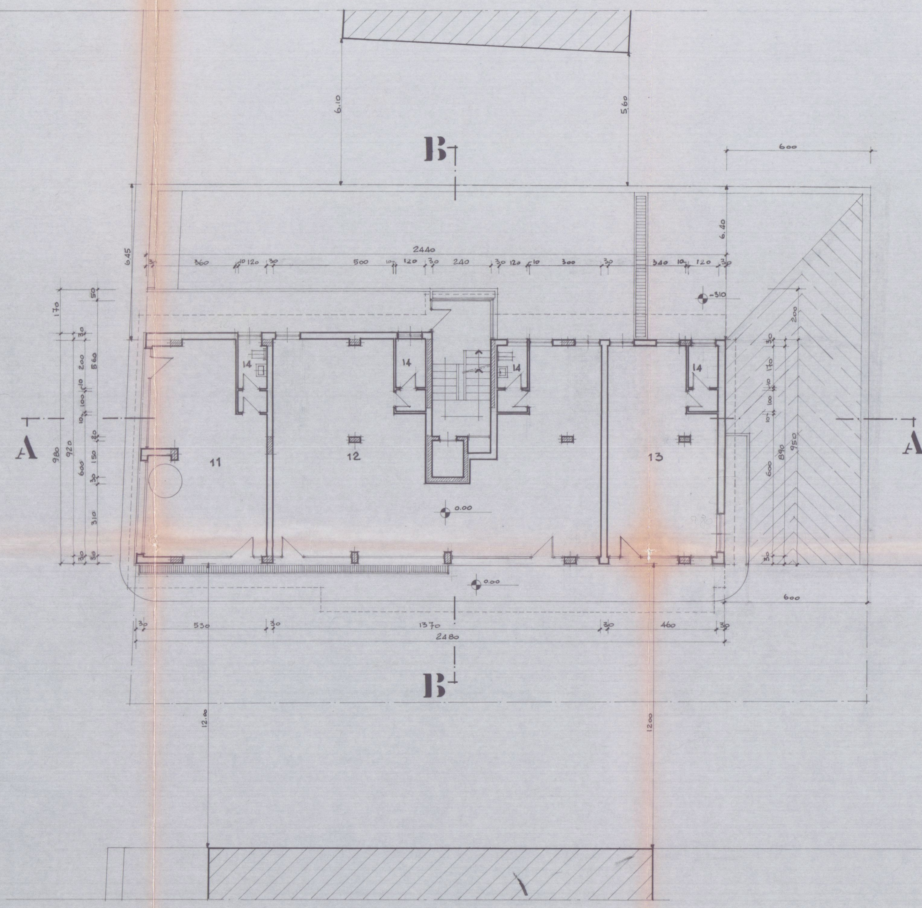
PIANTA PIANO TERRENO
