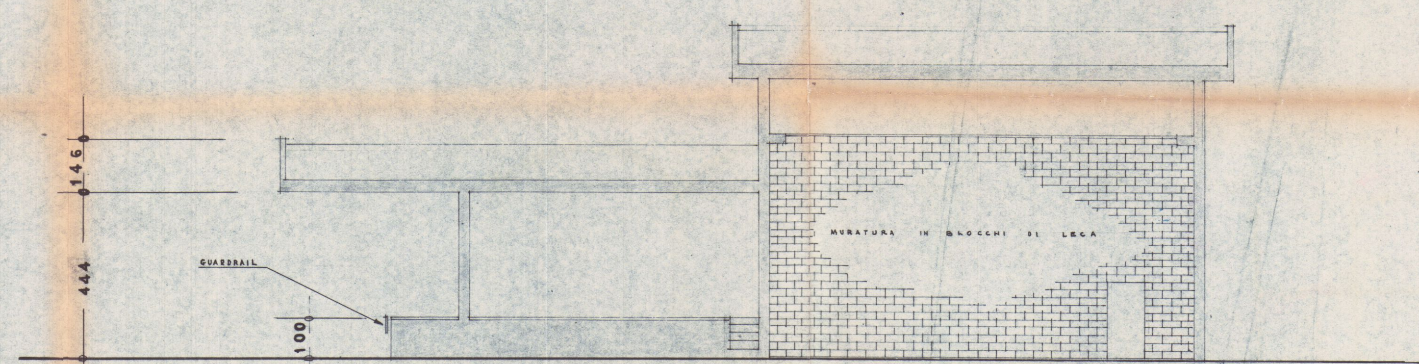
FIANCO NORD_EST
