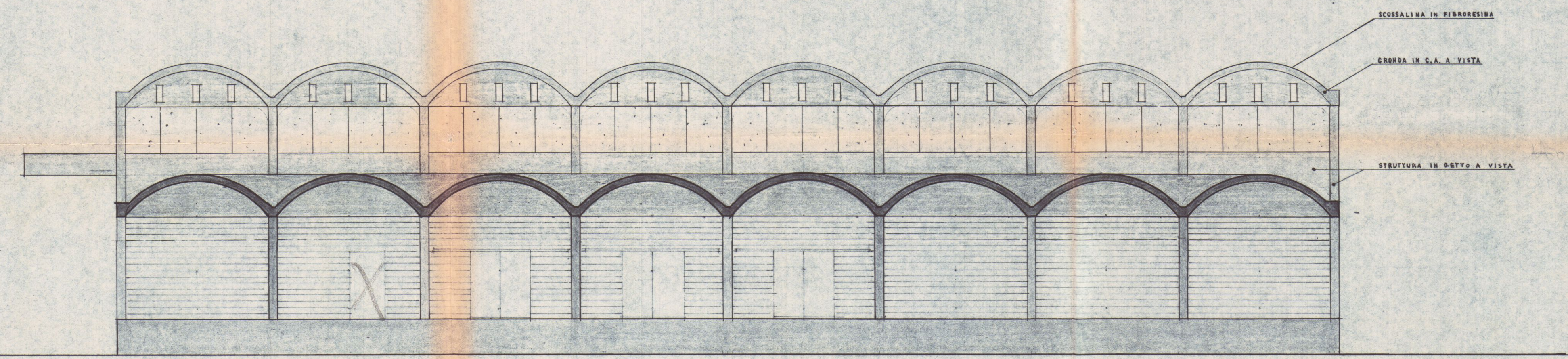
PROSPETTO SUD_EST
