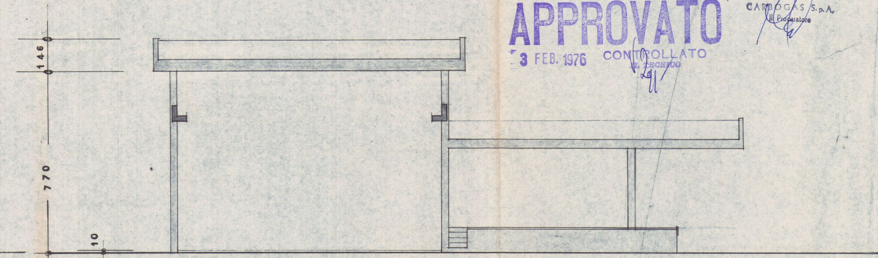
FIANCO SUD_OVEST
