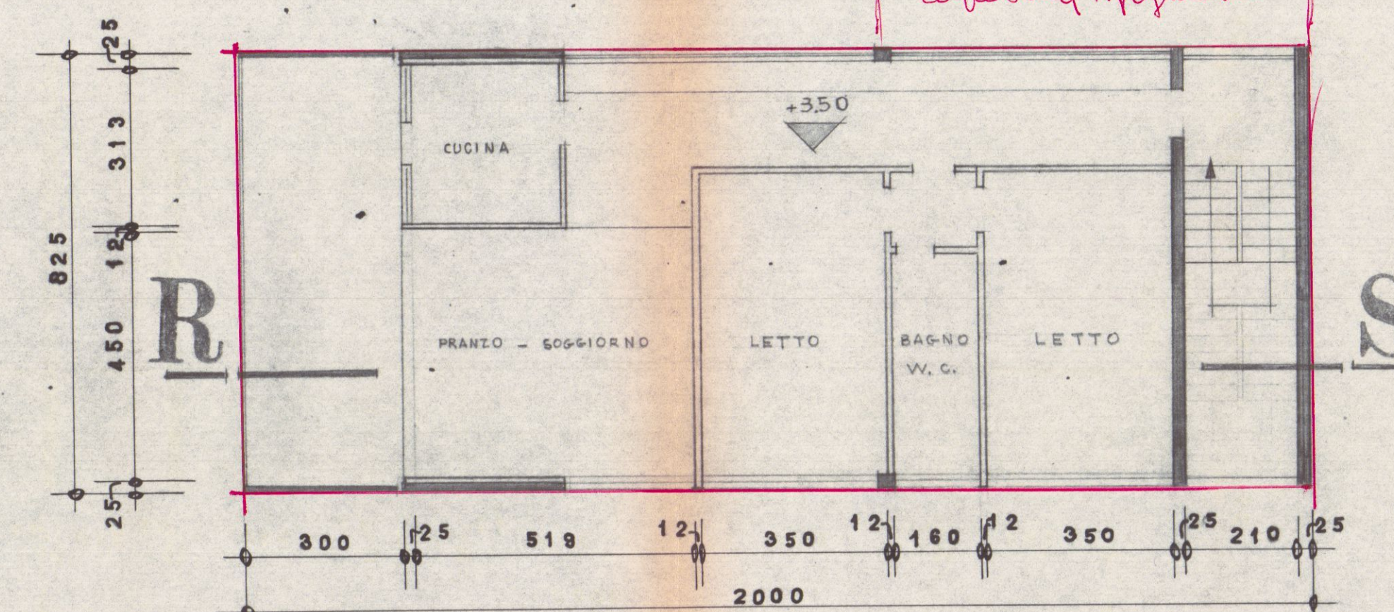
APPARTAMENTO CUSTODE SCALA 1:100 FABBRICATO B PIANO SUPERIORE
