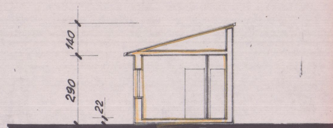
"SEZ. AA"
