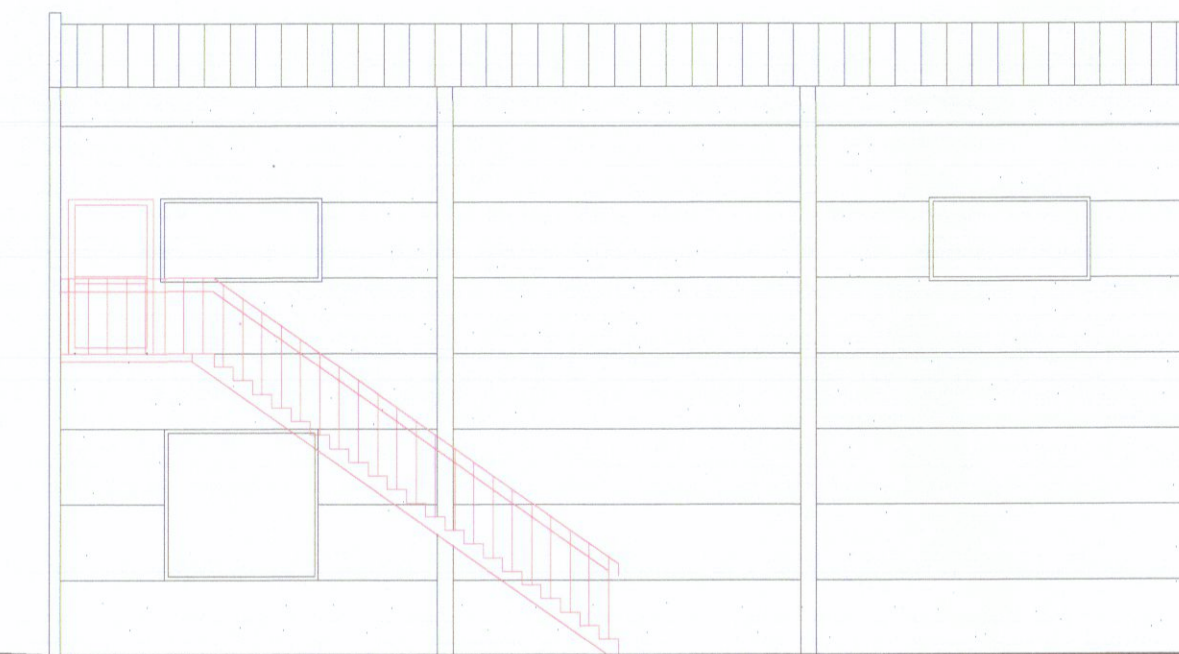
PROSPETTO-SUD
