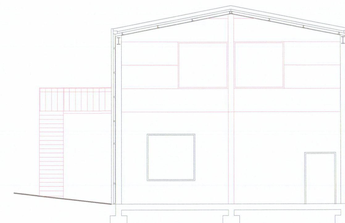
SEZIONE a-a'
