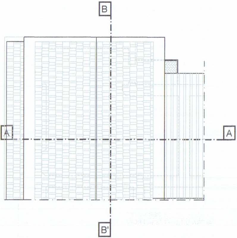
PIANTA PIANO COPERTURA scala 1.100
