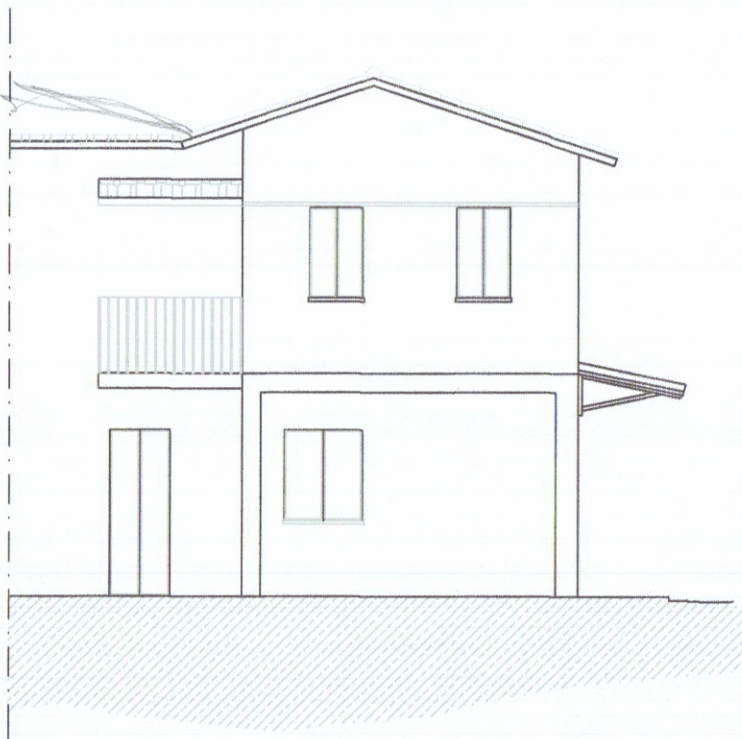
PROSPETTO PRINCIPALE scala 1.100
