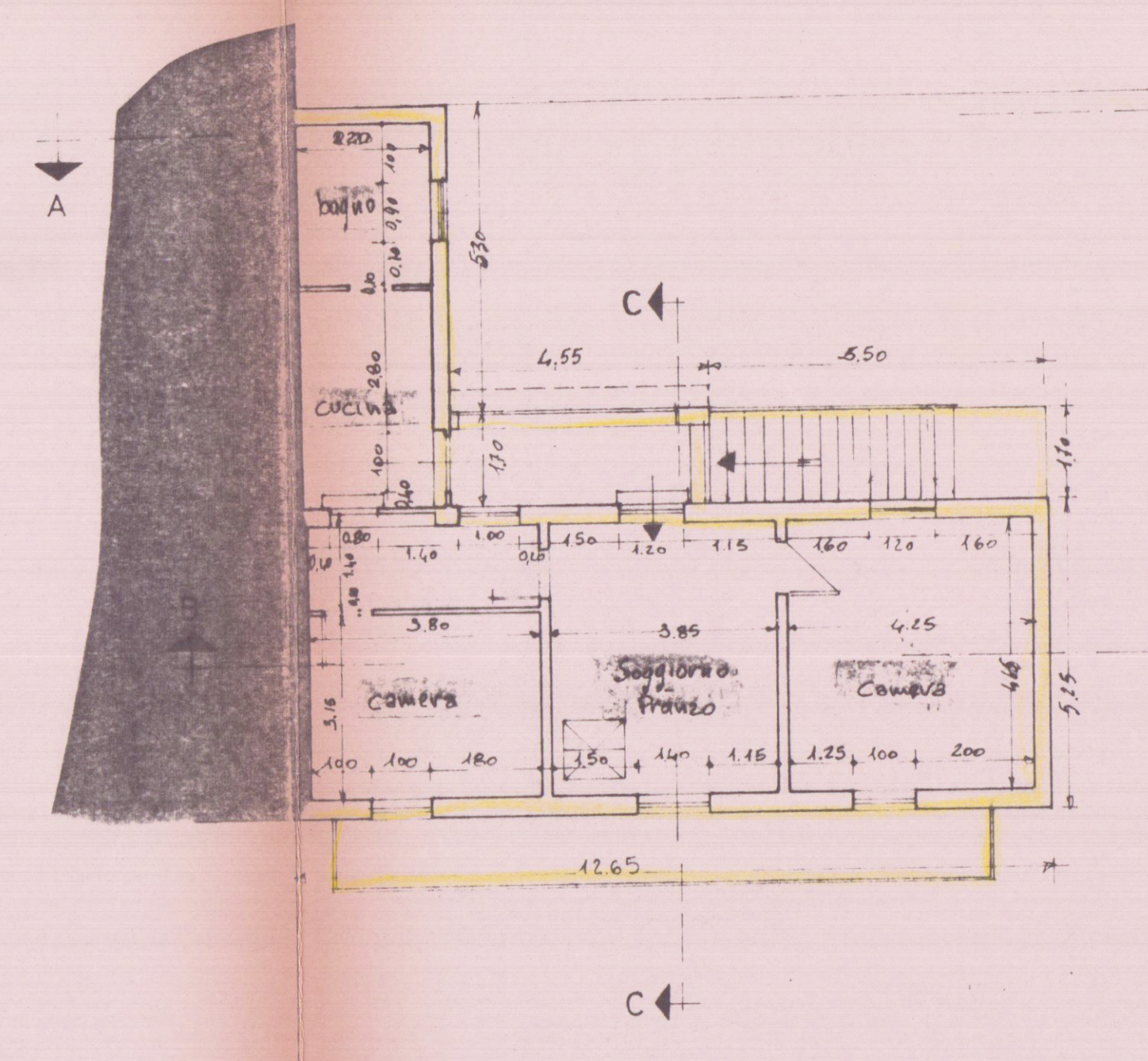
PIANO PRIMO
