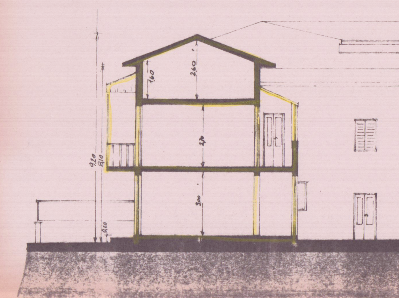
SEZIONE CC
