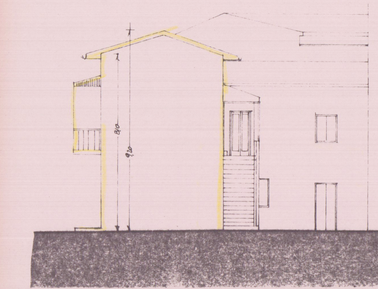
PROSPETTO LATERALE
