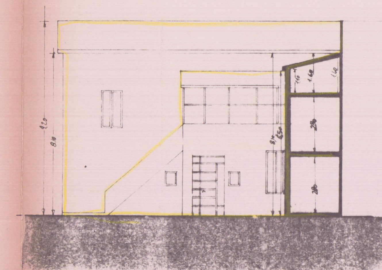
SEZIONE AA
