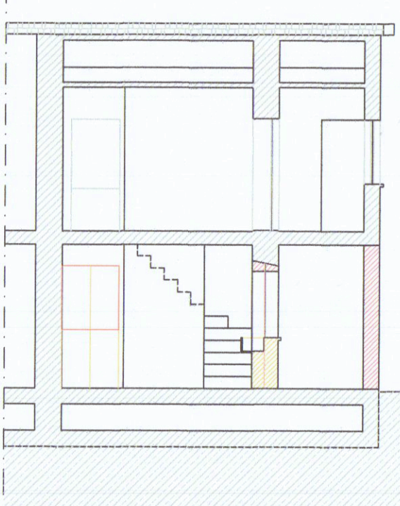
SEZIONE B-B' scala 1.100
