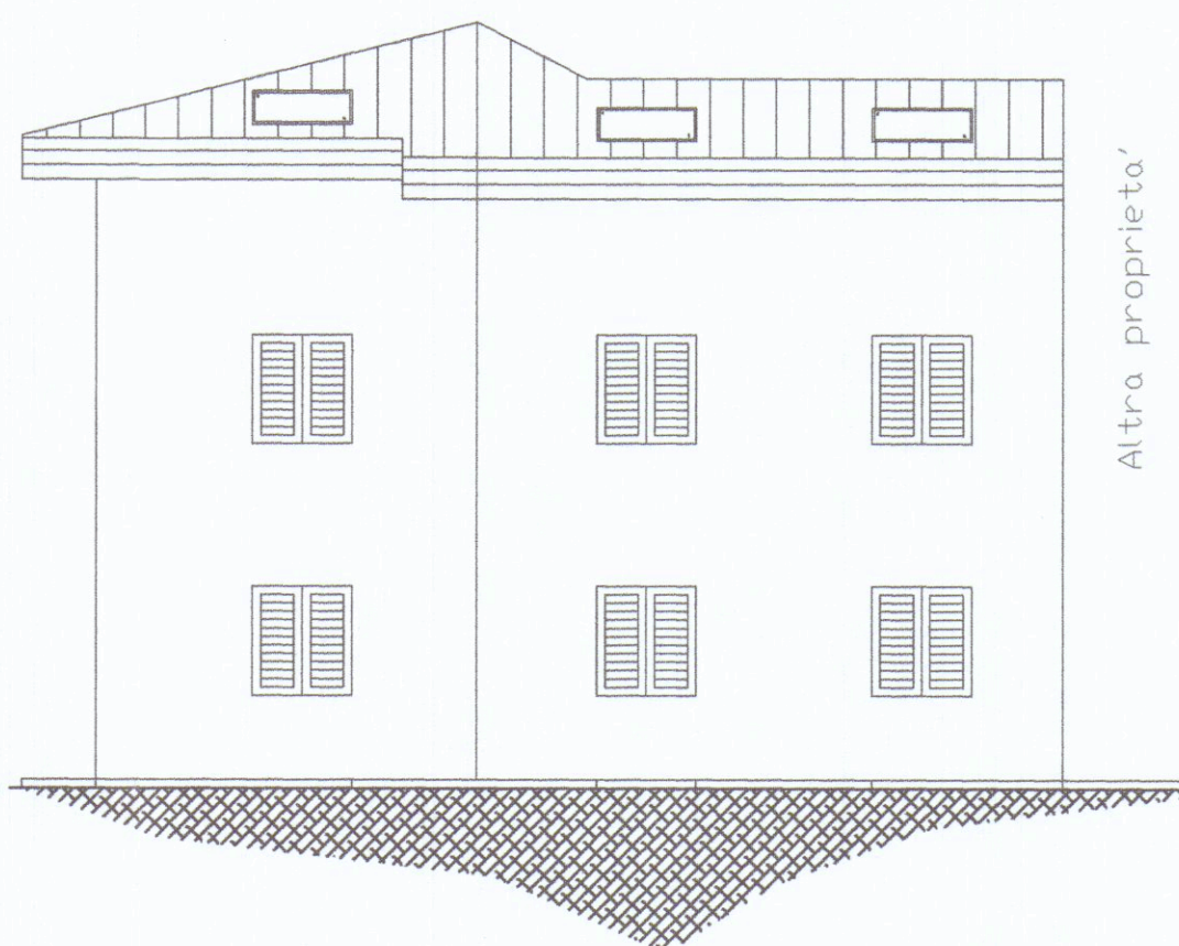
PROSPETTO NORD
