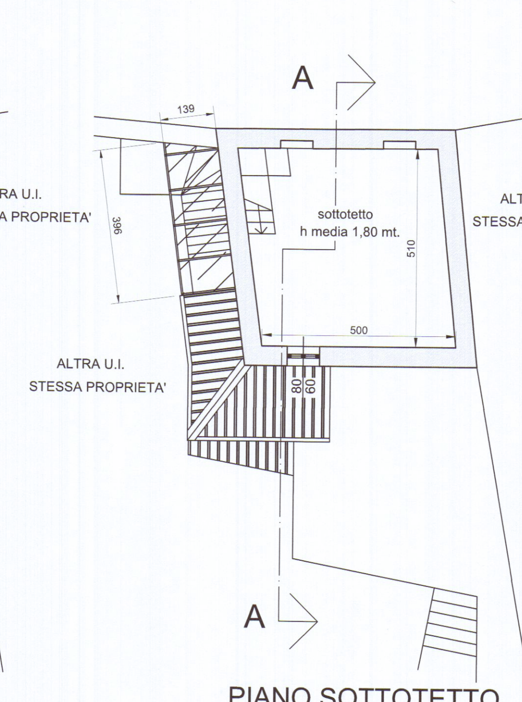
PIANO SOTTOTETTO
