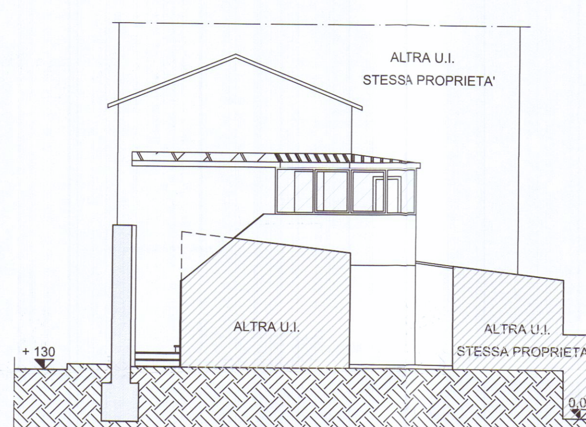
PROSPETTO OVEST
