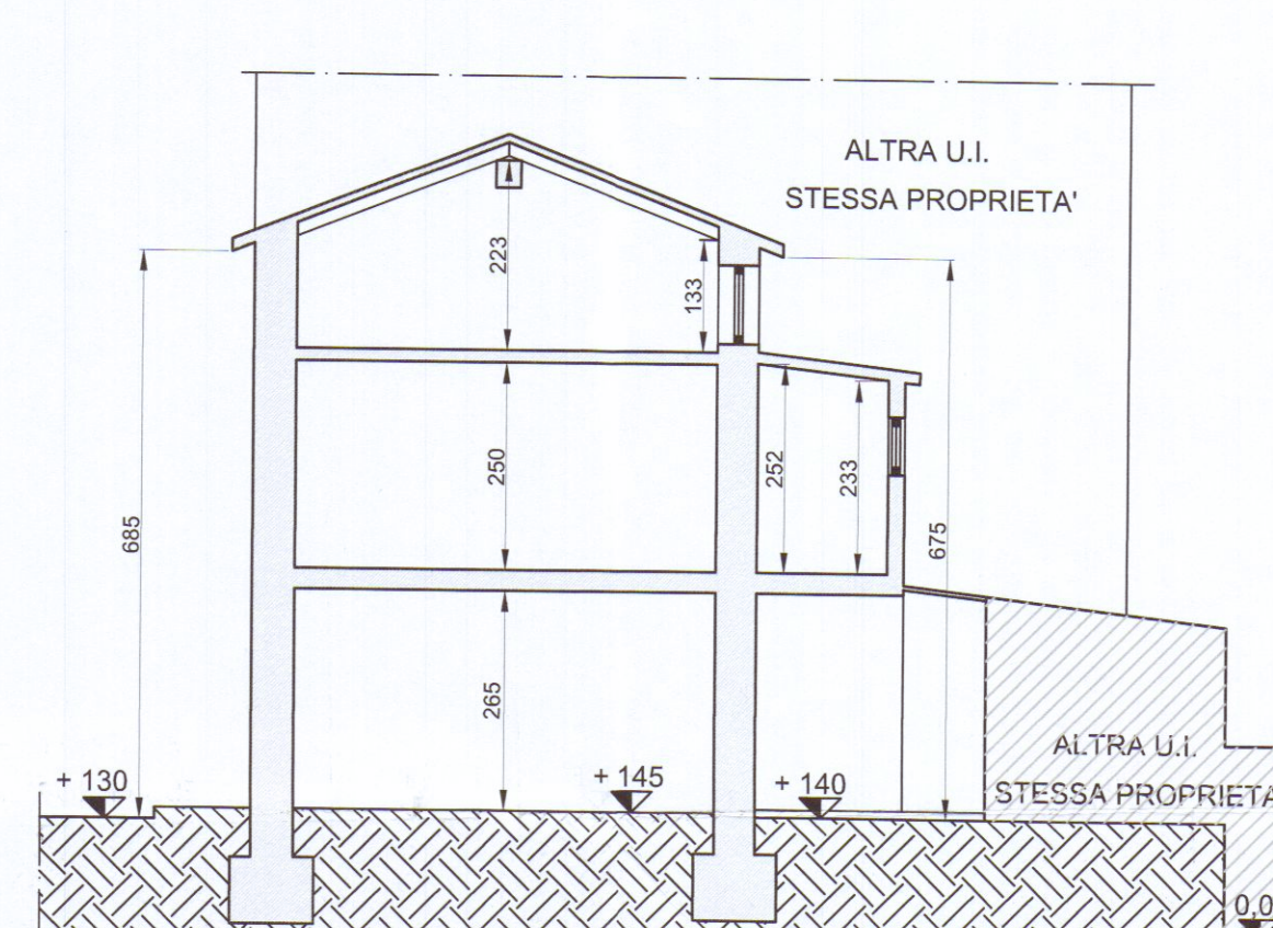
SEZIONE A-A
