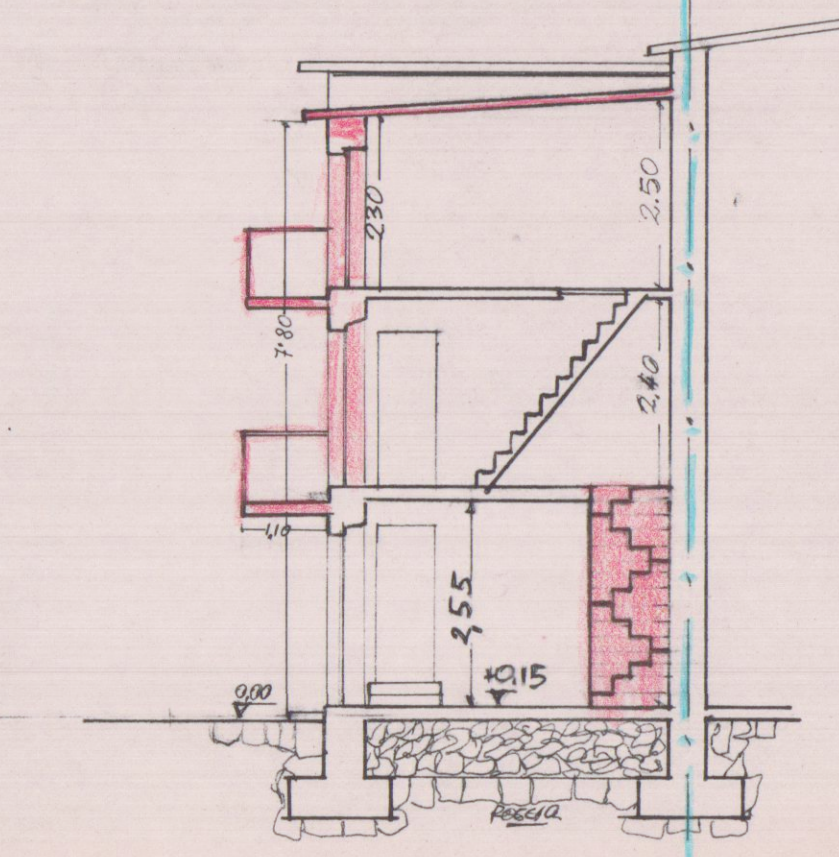
Sezione B-B
