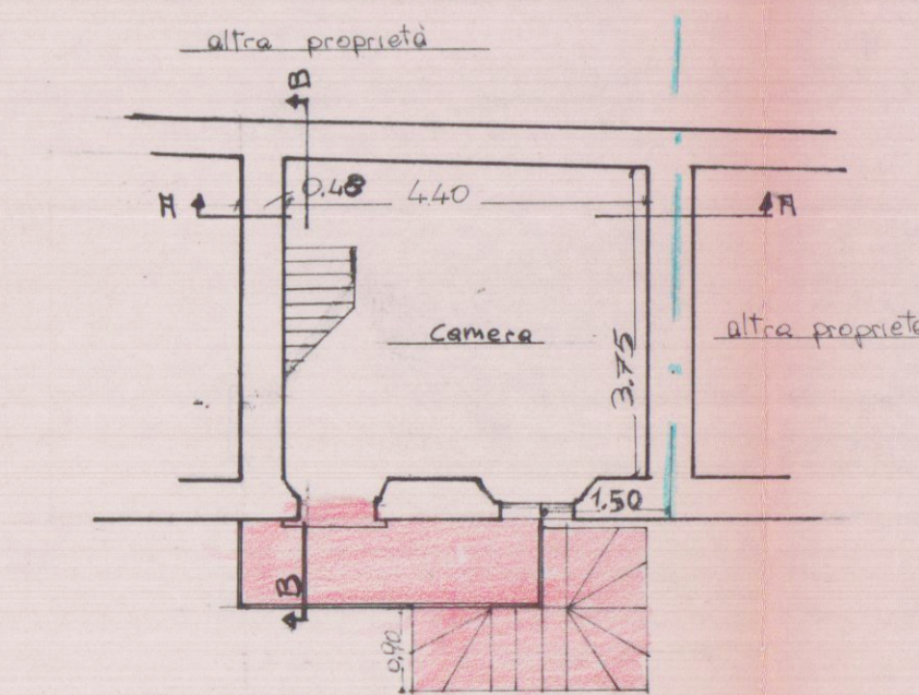
Piano secondo
