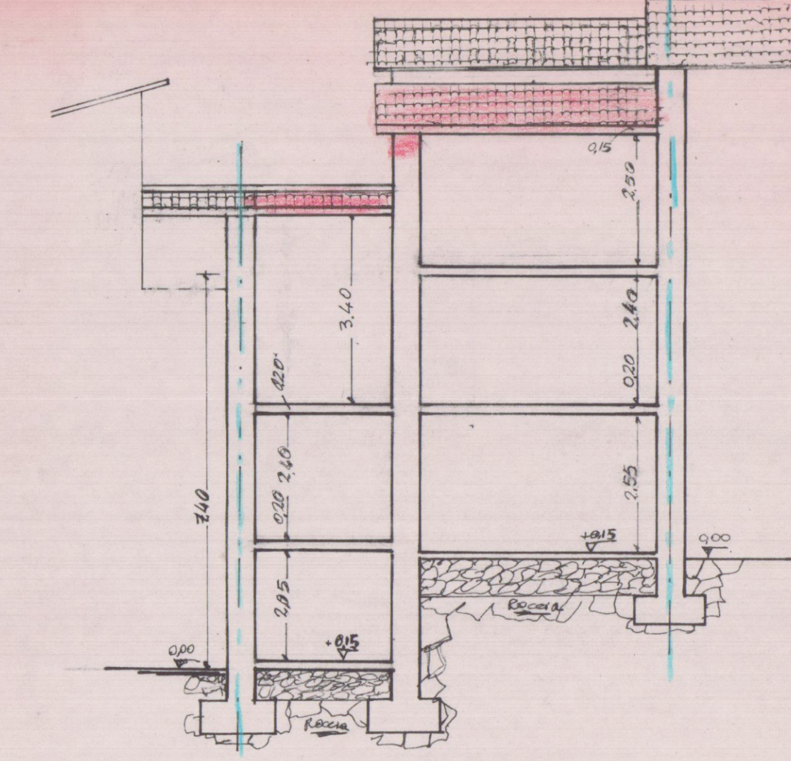
Sezione H-A
