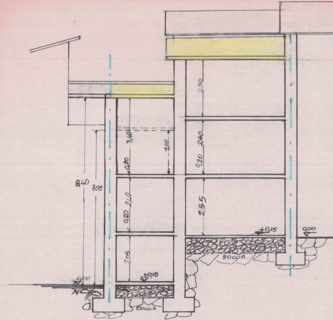
Sezione A-A
