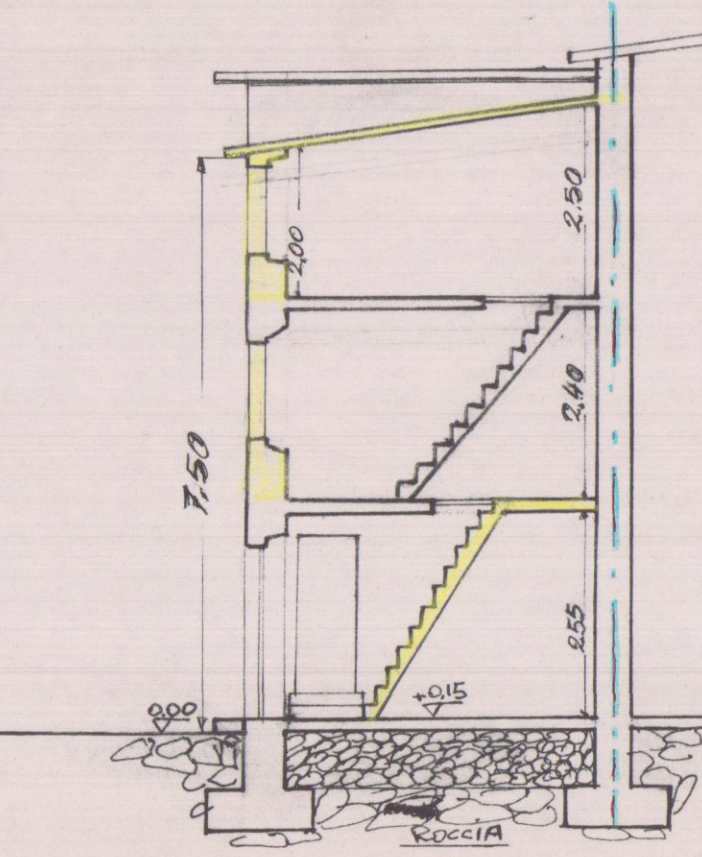
Sezione B-B
