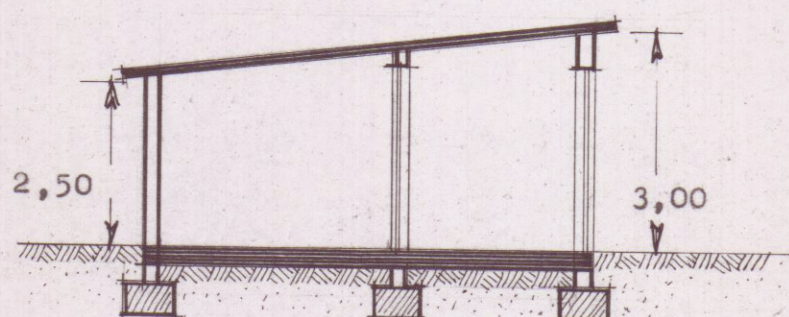
SEZIONE AB Fabbricato "B"
