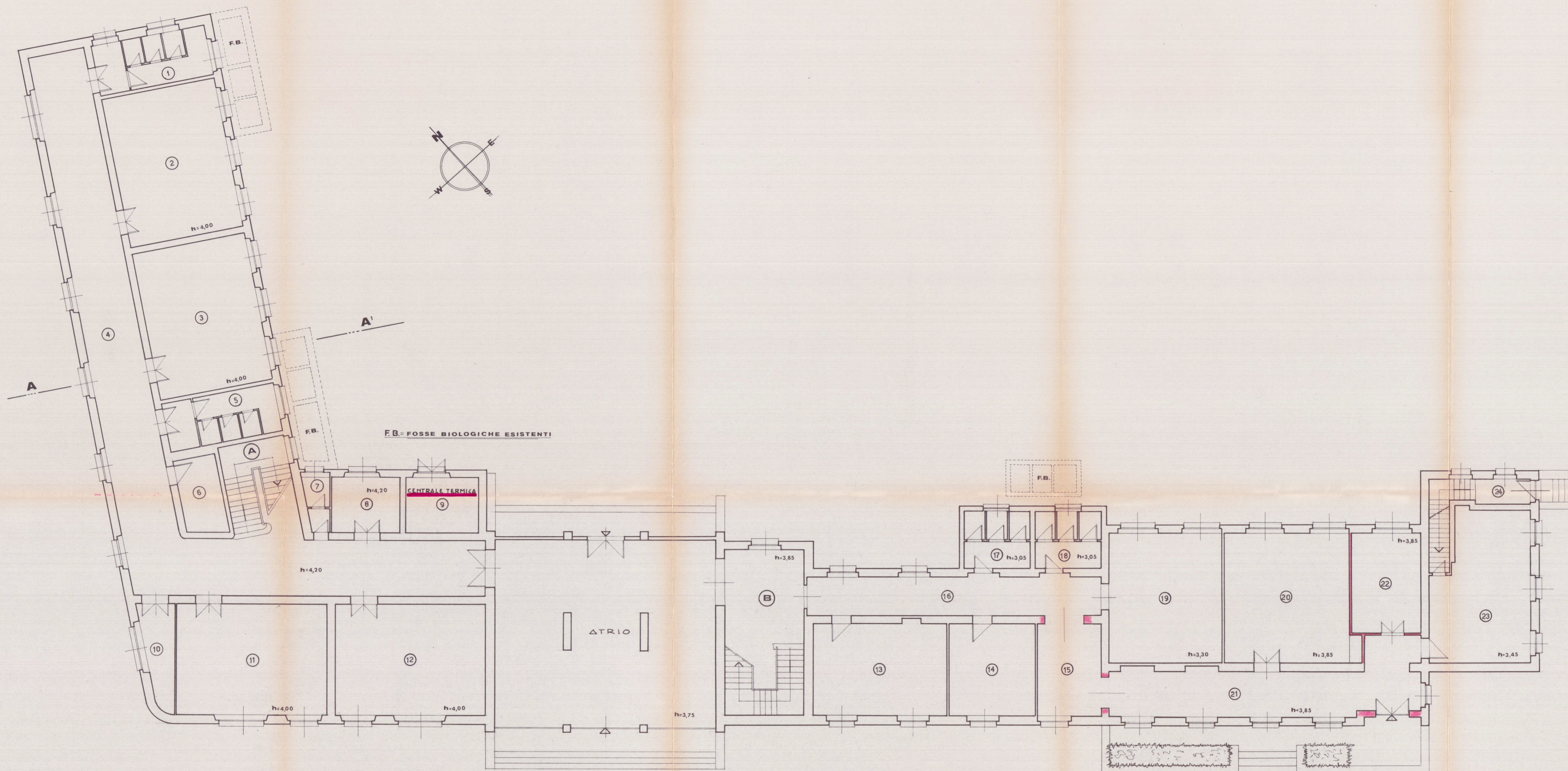
- PIANTE DEL PIANO RIALZATO - RAPP. 1:100 -
