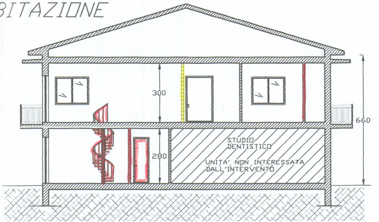
SEZIONE D-D
