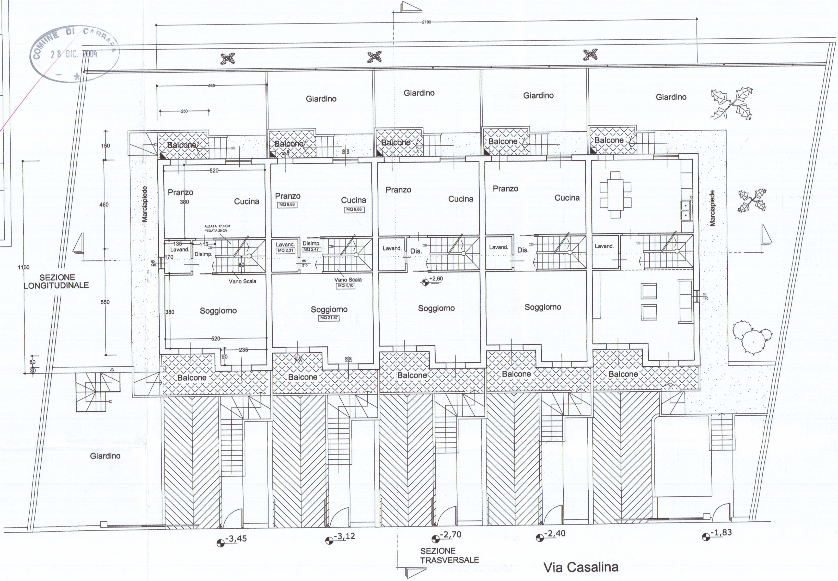
PIANTA PIANO RIALZATO
