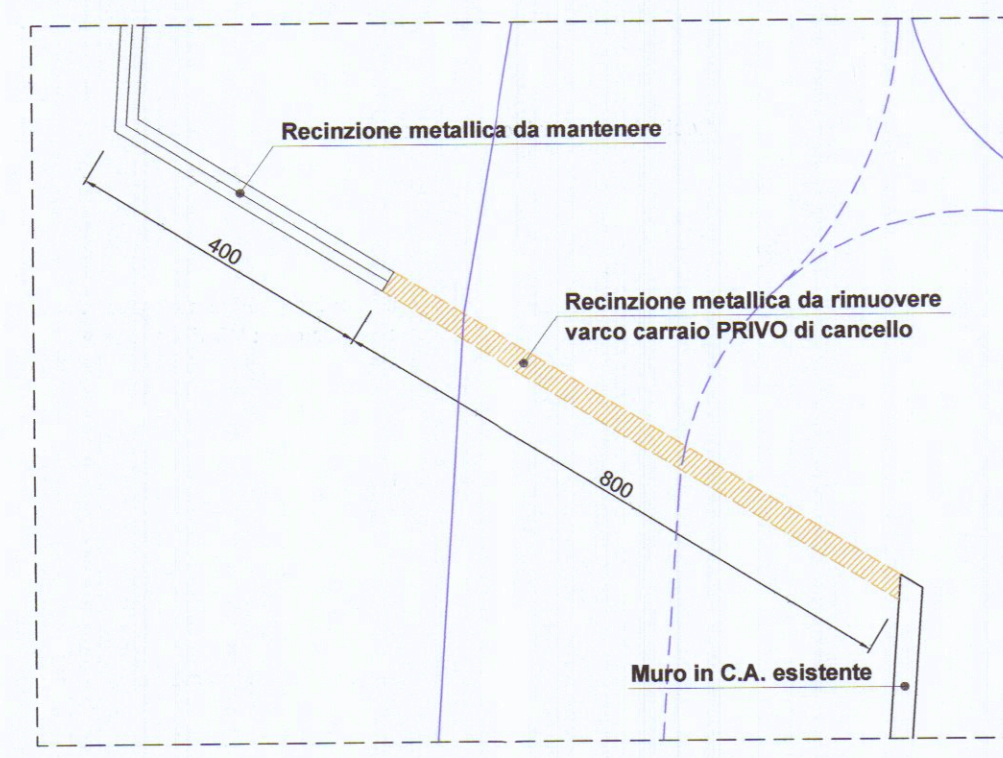
PARTICOLARE A - PIANTA NUOVO VARCO CARRAIO Scala 1:100
