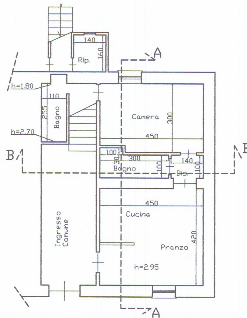
Pianta Piano Terra Cappellini
