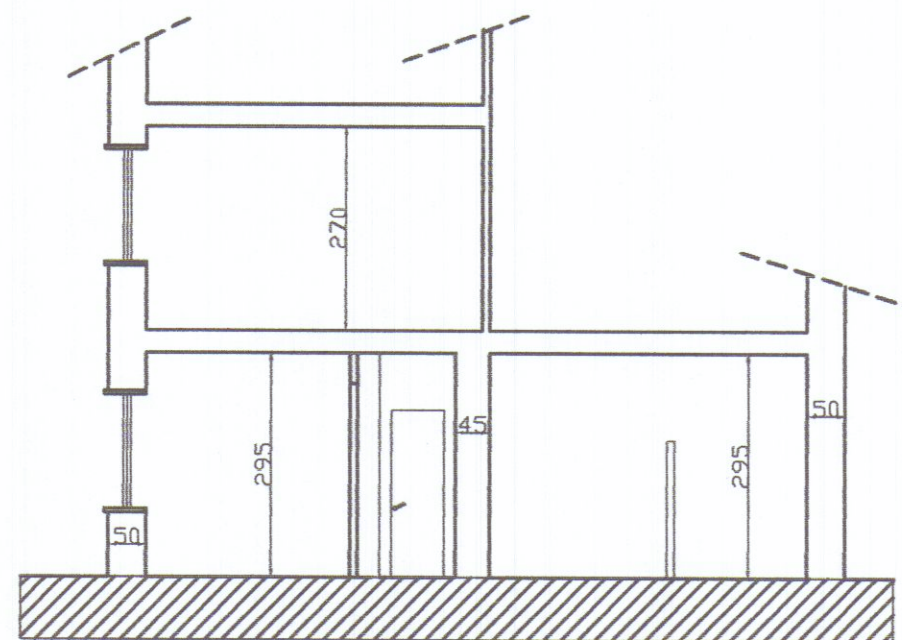
Sezione A-A
