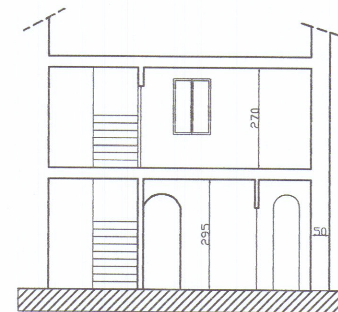
Sezione B-B
