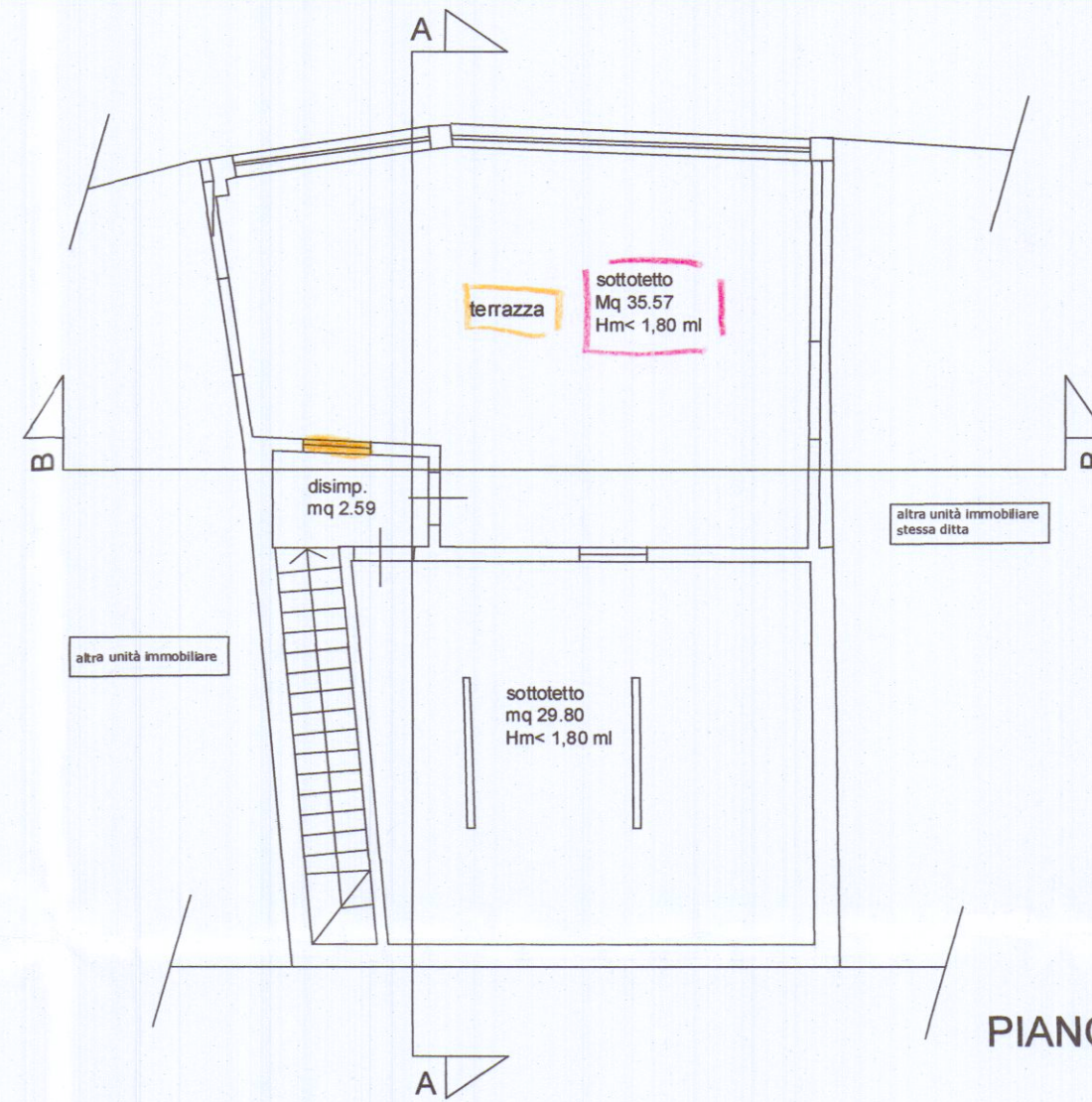
PIANO PRIMO
