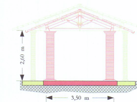
PROSPETTO NORD E SUD
