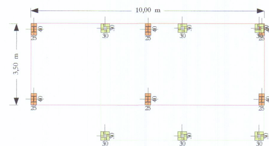
PIANTA
